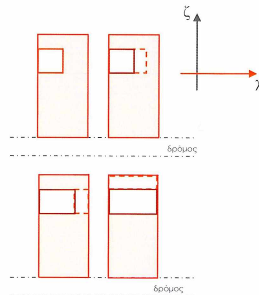
Εικόνα 139 Ανάπτυξη πυρήνα _Σχέση δομημένου-αδόμητου χώρου σε παραλληλόγραμμα στενομέτωπο οικόπεδο _Κάτοψη
