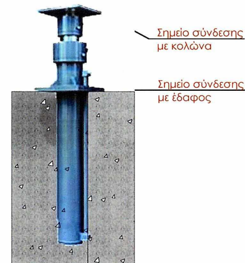
Εικόνα 159 Μπουτίλιες Ανύψωσης _Έδραση σε σκυρόδεμα [σημειακά στο οικόπεδο]
