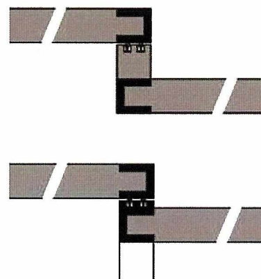
Εικόνα 160β Τρόπος Κύλισης Δωματίων _Τομή
