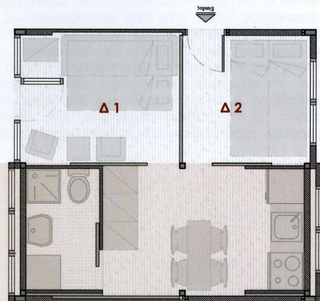
Εικόνα 145 Επέκταση Άνω πλευράς Oblong_Κάτοψη 26,5 τ.μ. συνολικά
