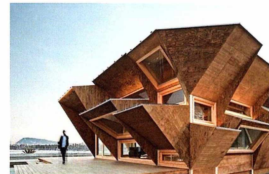
Εικόνα 198 Περίπτερο
