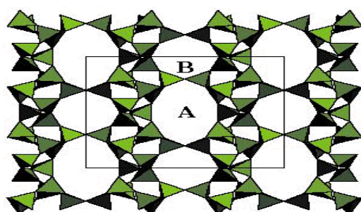
Εικόνα 1.2.2.1.2.2: Βασική δομή του κλινοπιτιλόλιθου (Κάτσου, 2011).
