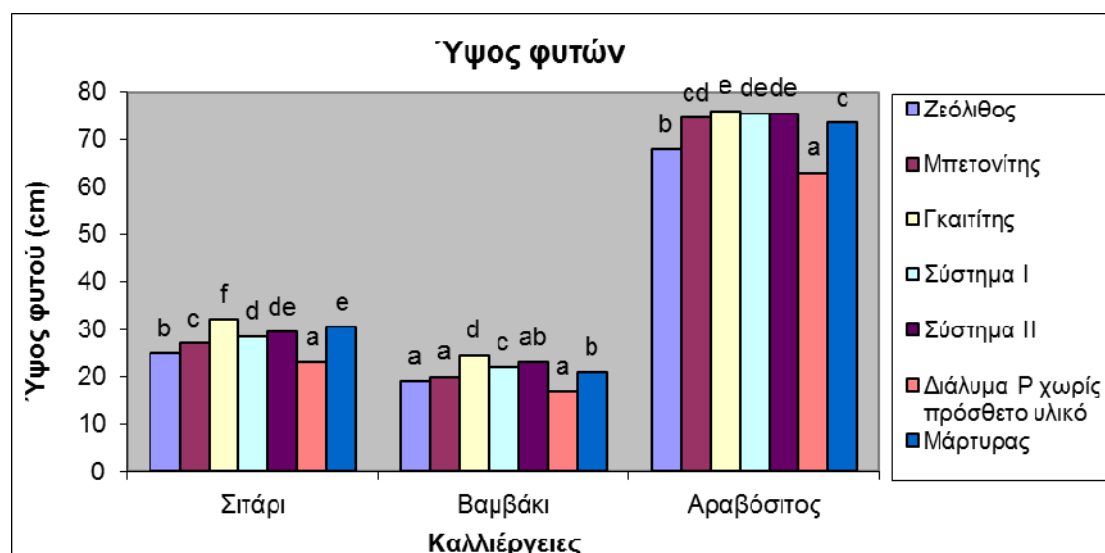
Σχήμα 3.2.1.1.1: Ύψος φυτών σιταριού, βαμβακιού και αραβοσίτου, που αναπτύχθηκαν σε έδαφος επιβαρυνμένο ή μη με φώσφορο και εφοδιασμένο ή μη, με τα υλικά Ζ, Β, Γ, Σ I και Σ II.
