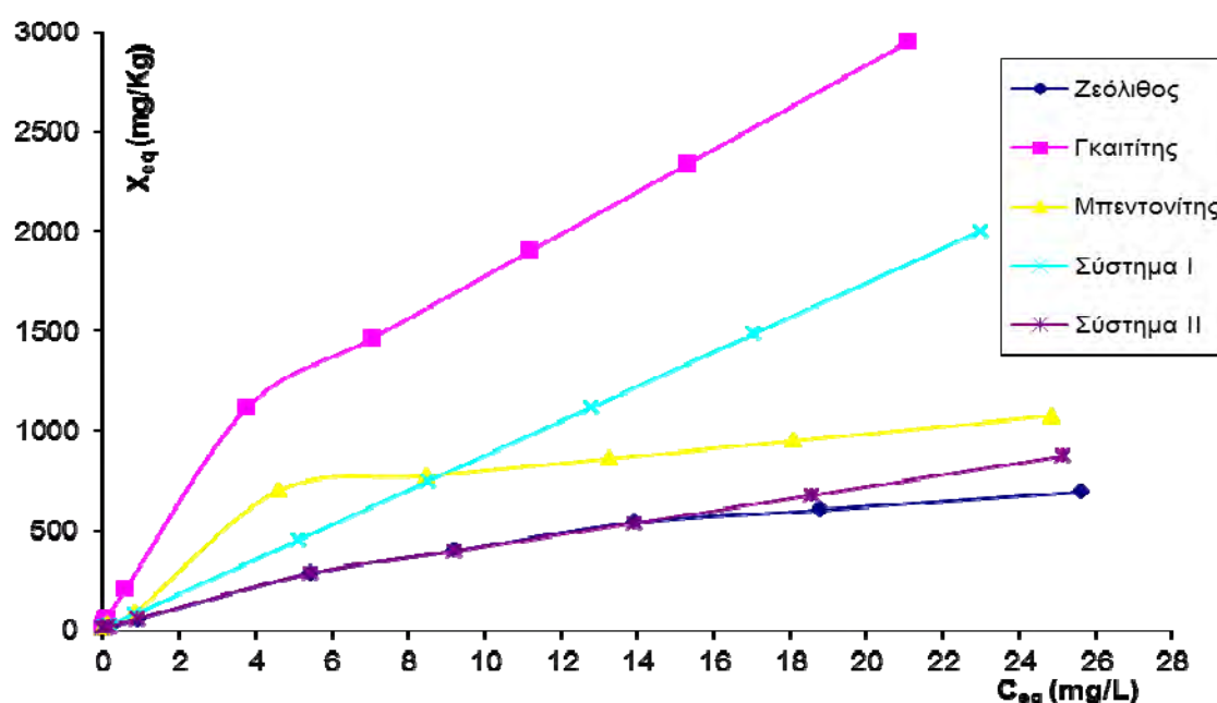
Σχήμα 3.1.1.1: Η προσρόφηση του φωσφόρου από υδατικά διαλύματα στα οποία έχουν προστεθεί τα υλικά ζεόλιθος, γκαιίτης, μπεντονίτης, σύστημα I και II, σε συνάρτηση με την συγκέντρωση ισορροπίας του φωσφόρου.
