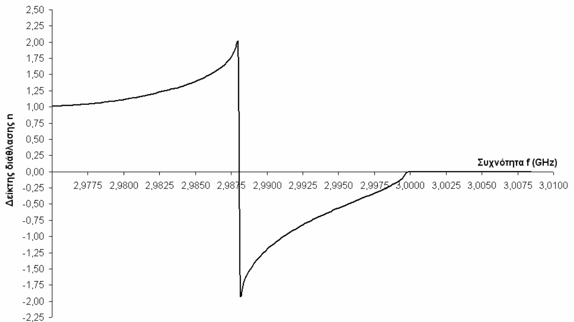
Σχήμα 5.9: Δείκτης διάθλασης της δομής για \epsilon_s = 150 , r_1 = 4.1 mm, r_2 = 5.8 mm.
