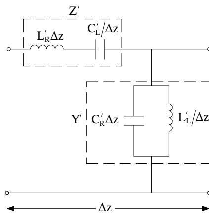
Σχήμα 1.10: Δομική μονάδα μεταυλικού
