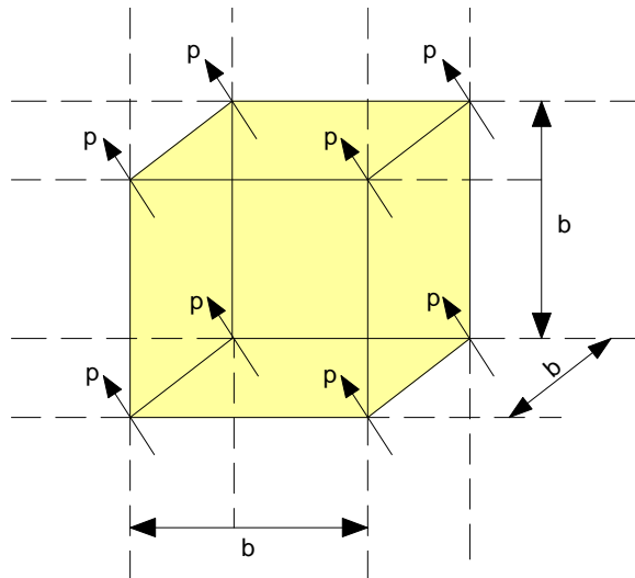
Σχήμα 3.2: Ηλεκτρικά δίπολα σε απλό κυβικό πλέγμα
