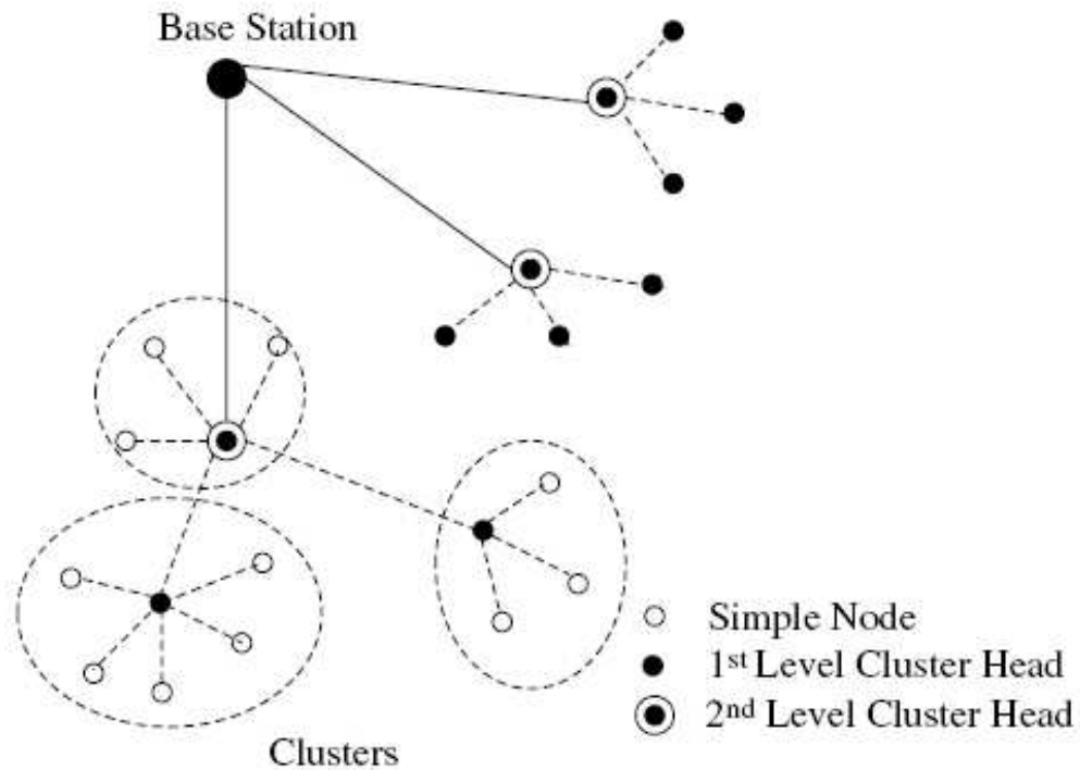
Εικόνα 29 - Hierarchical Clustering in TEEN and APTEEN
