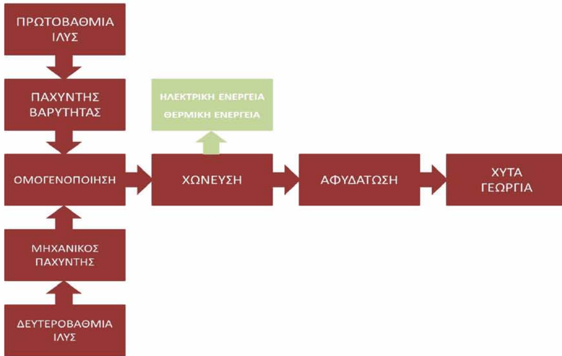
Σχήμα 4.2 : Επεξεργασία Ιλύος
