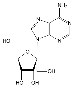
Psicofuranin
