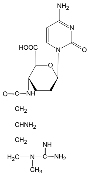
Blasticidin S
