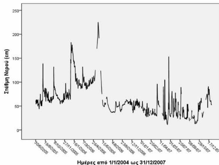
Σχήμα 3.47: Η χρονοσειρά της παραμέτρου στάθμη νερού στον Π.Σ. Νέστο.
