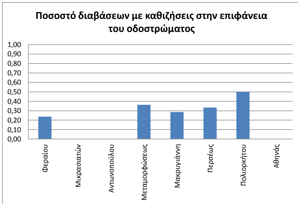
Σχήμα 3. 14: Ποσοστό διαβάσεων με καθιζήσεις στην επιφάνεια του οδοστρώματος
