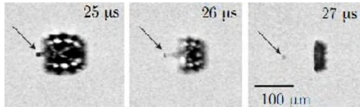
Σχήμα 4.3 Λεπτομέρειες της εξέλιξης του jet την στιγμή της σύγκρουσης των αντίθετων τοιχωμάτων της φυσαλίδας για 100μl.
