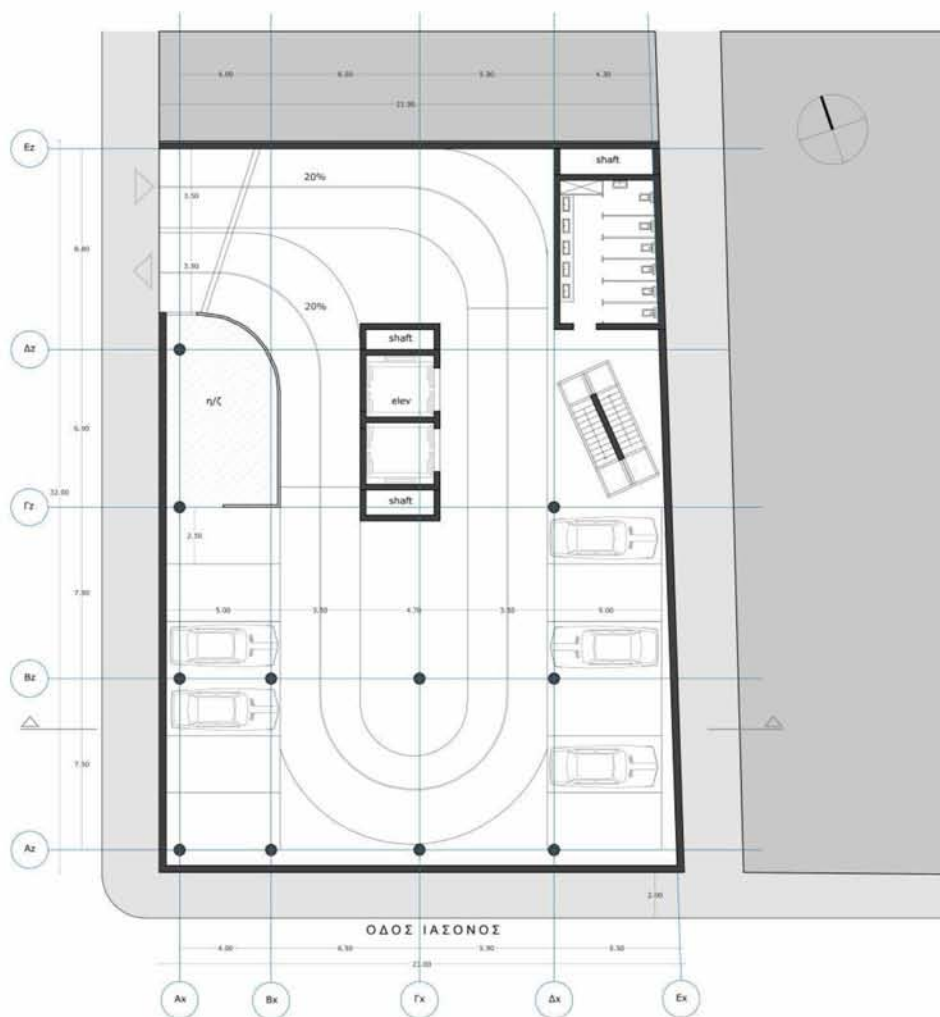
Εικόνα 25 κατόψη υπογείου
