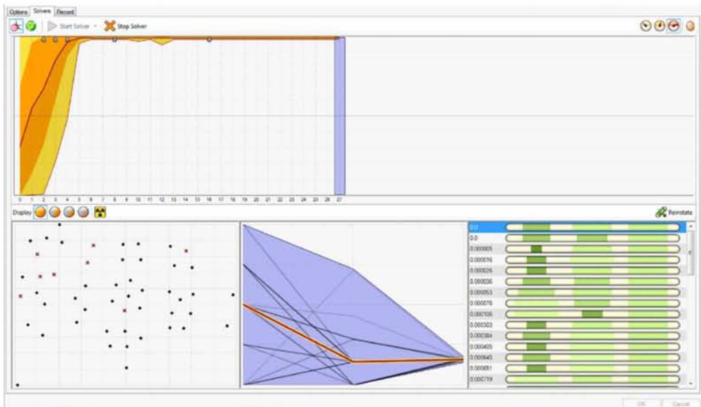
Εικόνα 21 Galapagos editor
