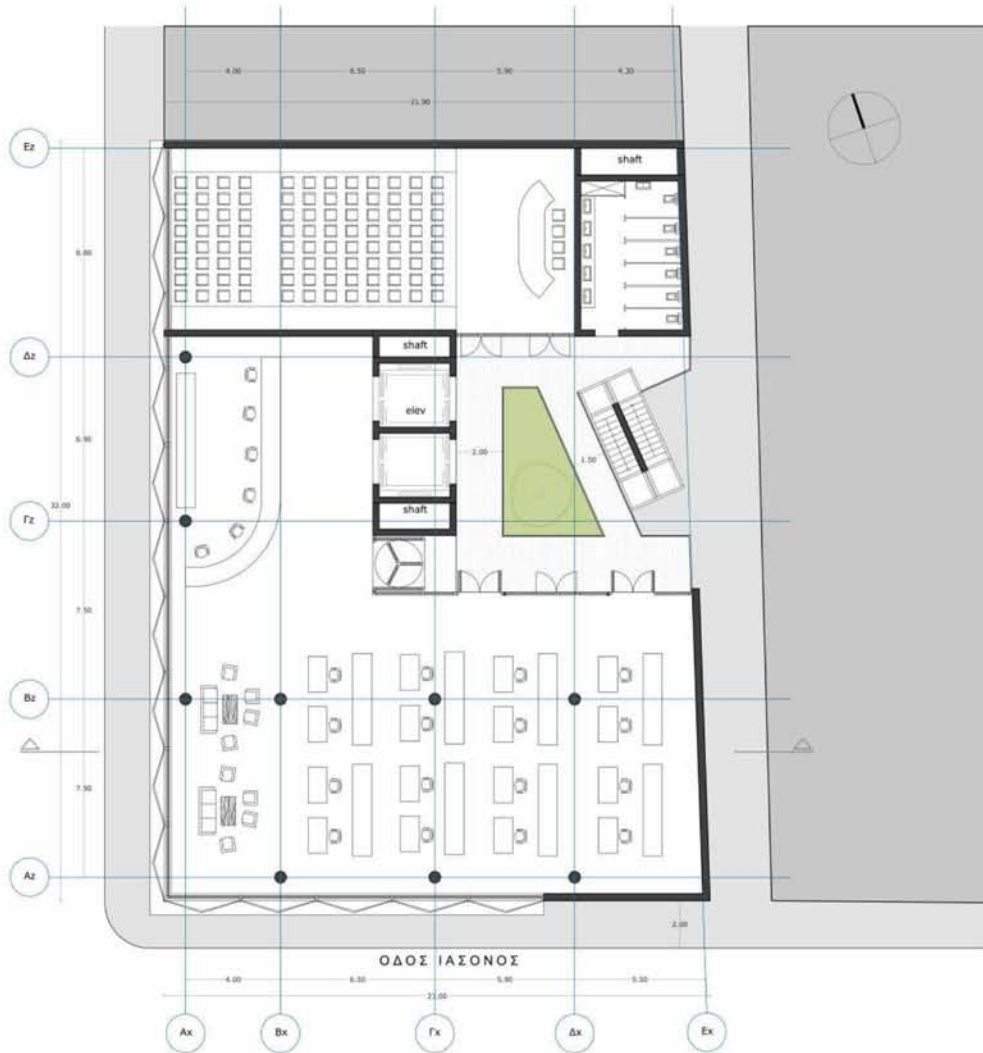
Εικόνα 27 κατόψη α ορόφου
