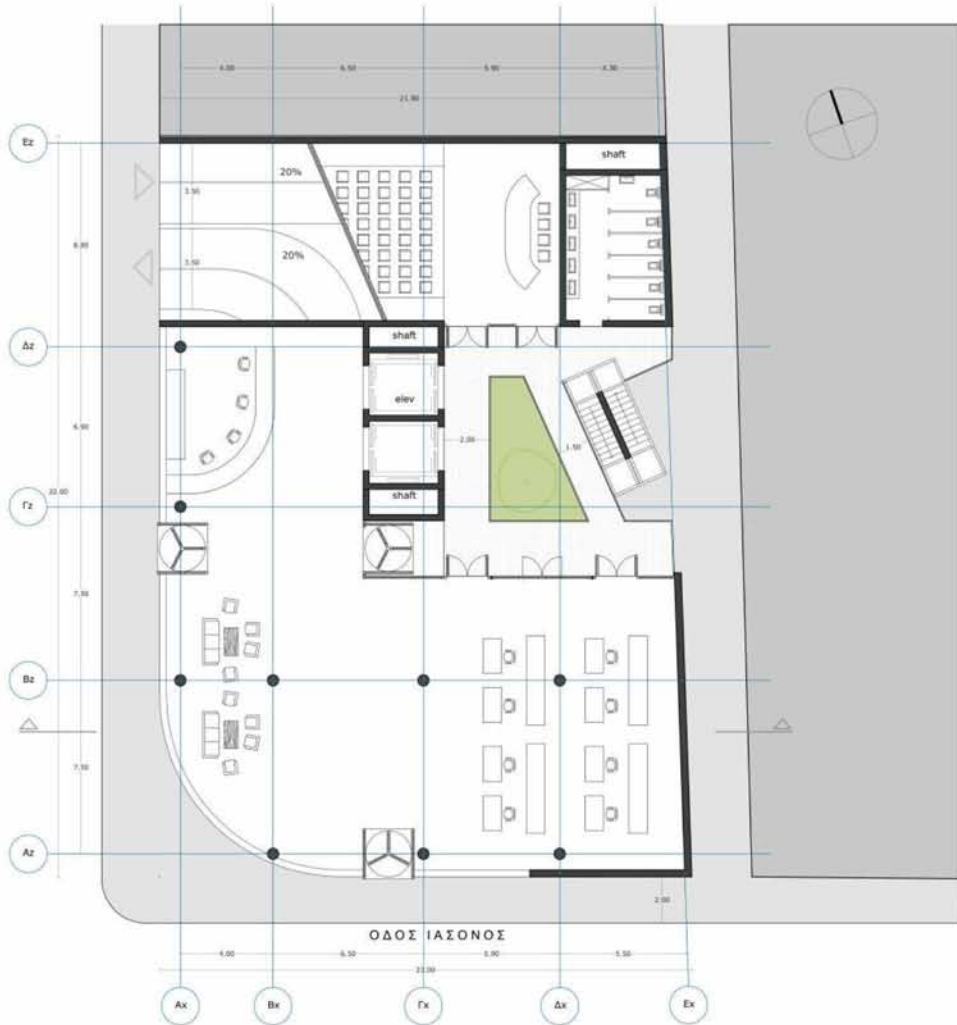
Εικόνα 26 κάτοψη ισογείου
