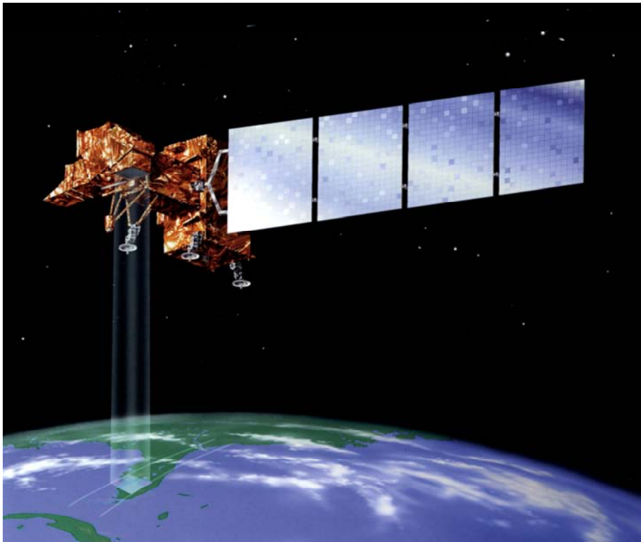
Εικόνα 2. Δορυφόρος Landsat
