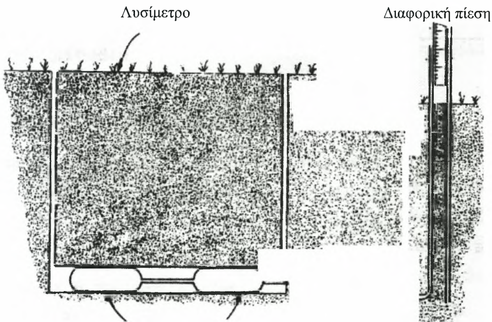
Σχήμα 3.1 / Ένα τυπικό Λυσίμετρο (Λυσίμετρο υδραυλικού τύπου)
