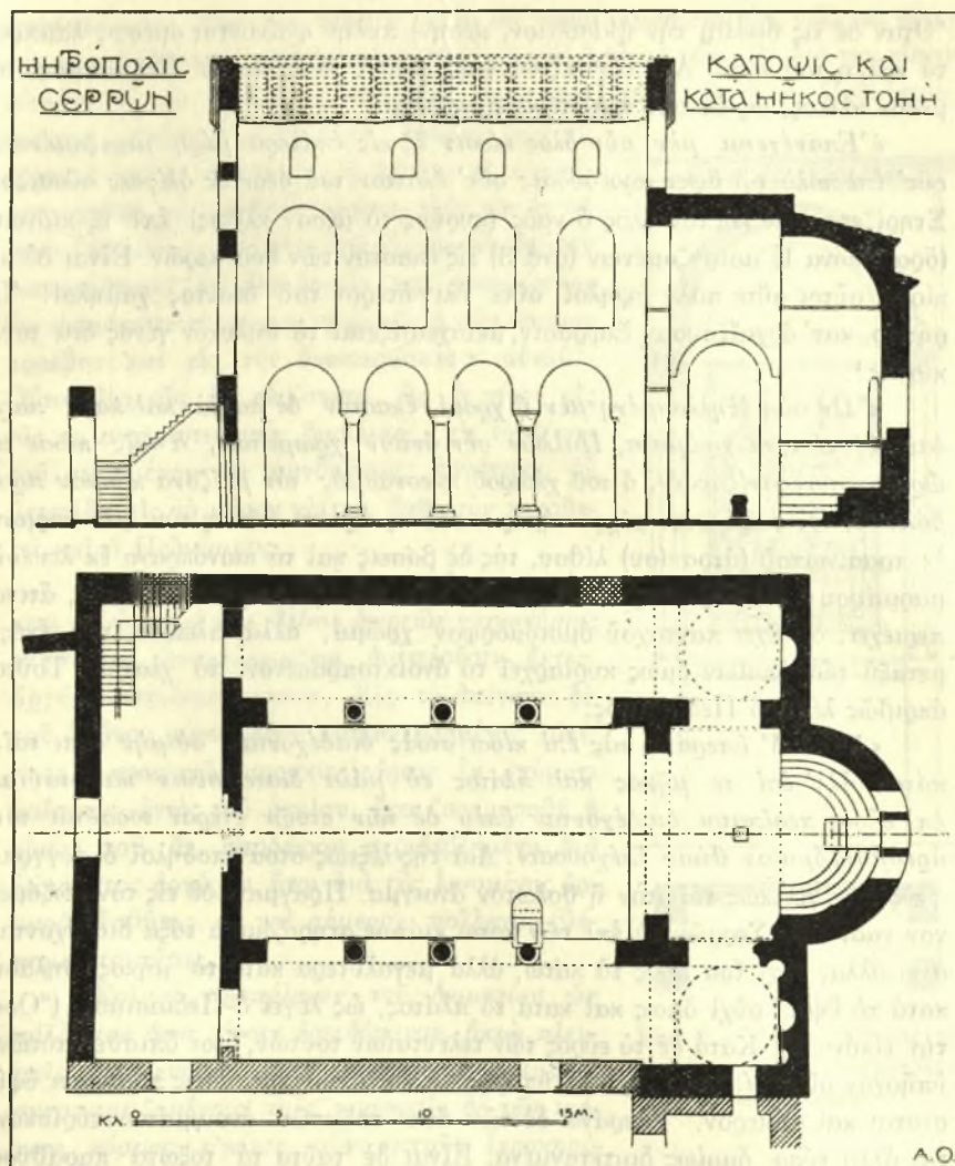
Εἰκ. 1.—Κάτοψις καὶ κατὰ μῆκος τομὴ τῆς Μητροπόλεως τῶν Σερρῶν (παρούσα κατάστασις).
