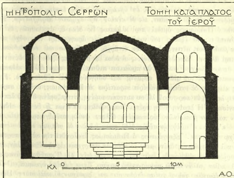
Εἰκ. 6.—Τομὴ κατὰ πλάτος τοῦ ἱεροῦ τῆς μητροπόλεος τῶν Σερρών.
