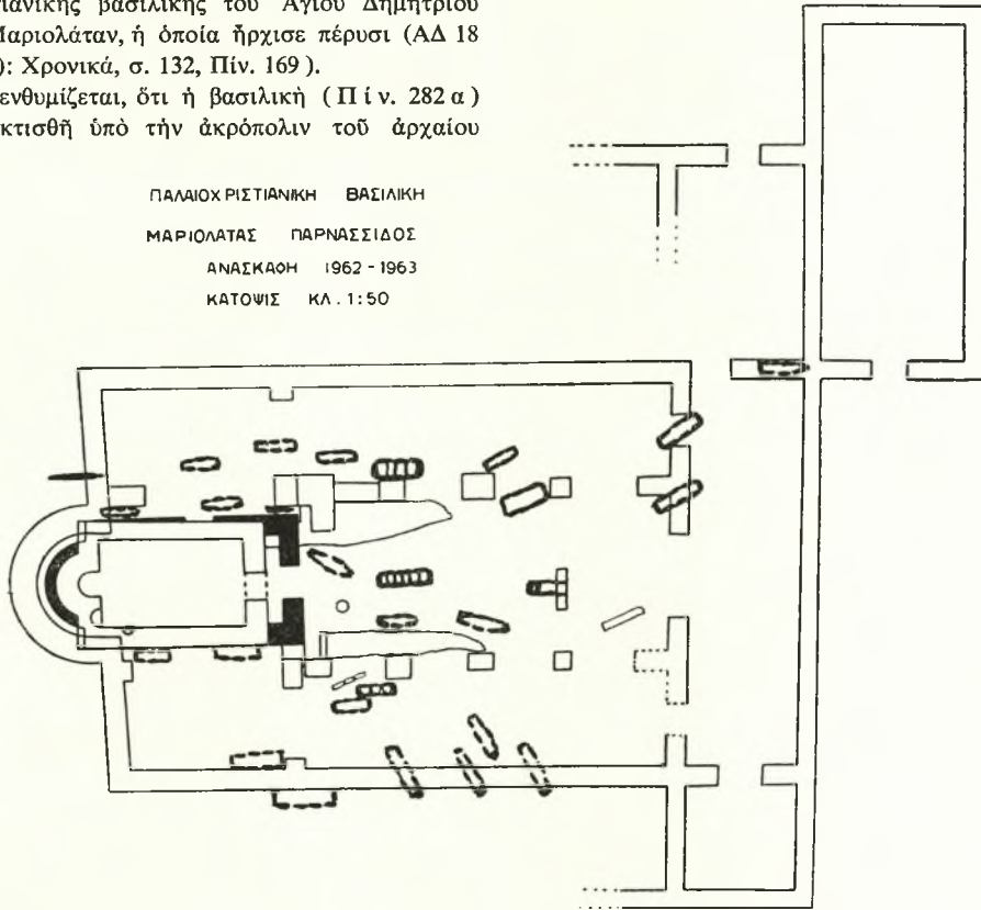
Σχέδ. 1. Μαρριολάτα. Κάτοψις βασιλικής
