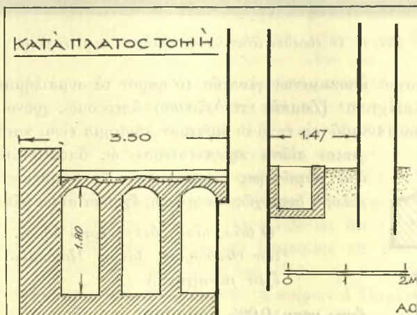
Εἰκ. 2. Κατακόρυφος τομὴ τῶν τάφων.
