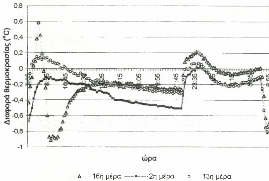
Σχήμα 3.3.6. Διαφορά θερμοκρασίας μεταξύ του αέρα του κλωβού στο ύψος των φυτών και του εξωτερικού αέρα \Delta T_{i_k - \theta_k} ( =T_{i_k} - T_{\theta_k} ) (°C) κατά τη διάρκεια του 24ώρου, τη δεύτερη, δέκατη τρίτη και δέκατη έκτη ημέρα της σκληραγώγησης.
