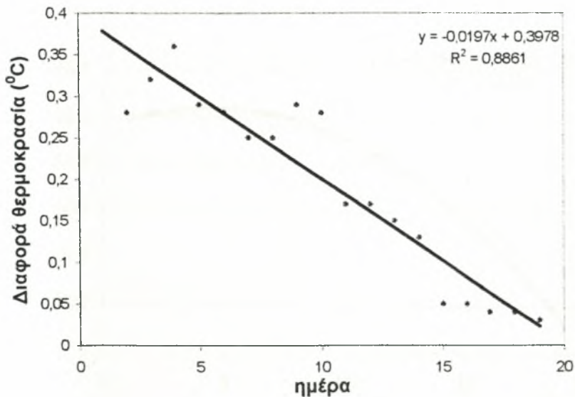
Σχήμα 3.3.5. Διαφορά θερμοκρασίας μεταξύ του αέρα του κλωβού στο ύψος των φυτών και του εξωτερικού αέρα \Delta T_{i_k - o_k} ( =T_{i_k} - T_{o_k} ) (°C) κατά τη διάρκεια της σκληραγώγησης των 19 ημερών.
