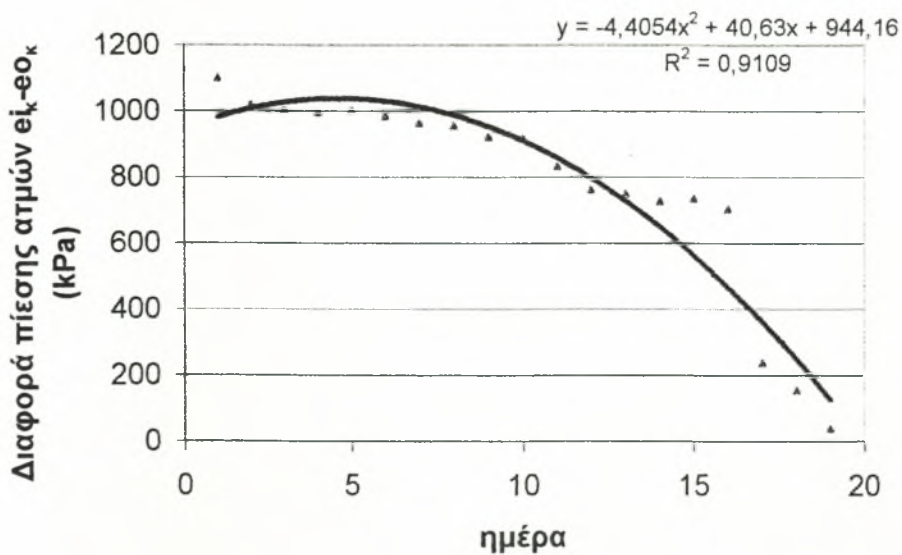
Σχήμα 3.3.7. Διαφορά μεταξύ πίεσης ατμών μεταξύ του αέρα του κλωβού και του αέρα του θαλάμου σκληραγώγησης \Delta \epsilon_{i_k} - \epsilon_{\theta_k} ( =\epsilon_{i_k} - \epsilon_{\theta_k} ) (kPa) τις 19 ημέρες εγκλιματισμού.
