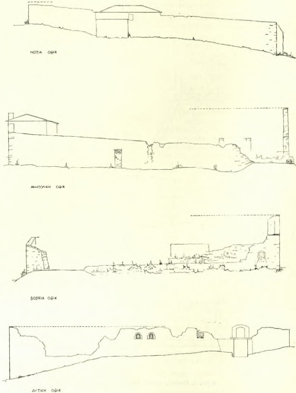
Σχέδ. 2. Μονὴ Πανάσσαρη. Σχεδιαστικὴ παράστασις τῶν τεσσάρων πλευρῶν, ὡς ἔχουν
