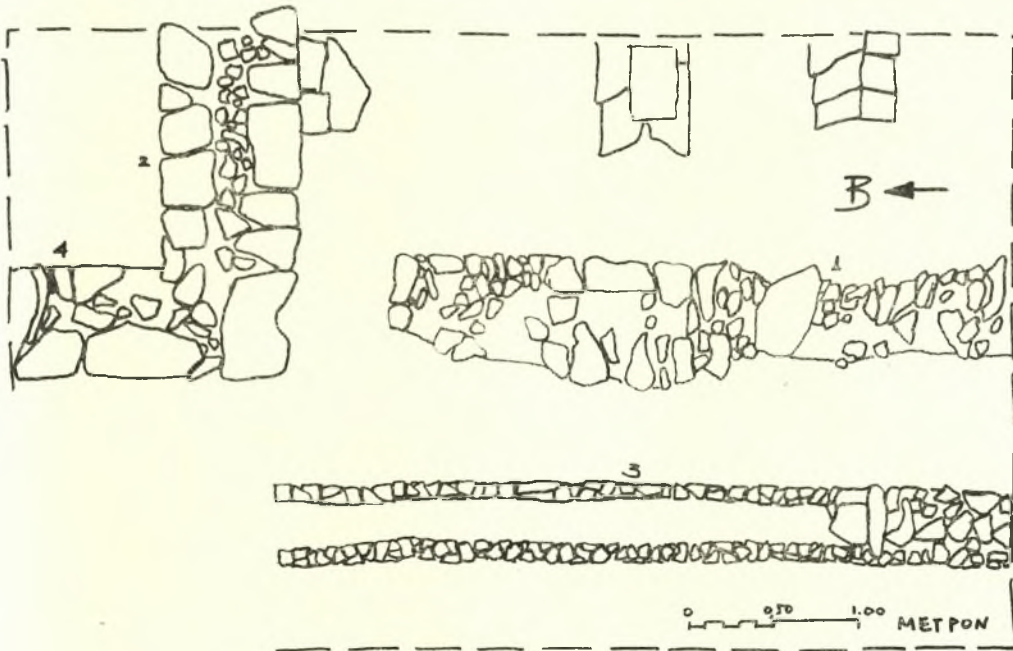
Σχέδ. 10. Θήβαι. Οικόπ. Όμμ. Όωάννου. Κάτωπις στρώματος Α
