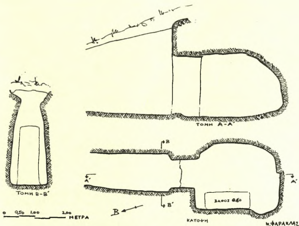
Σχέδ. 12. Θῆβαι. Κολωνάκι. Οἰκόπ. Μαρλάση. Κάτοψις καὶ τομαὶ θαλαμοειδοῦς τάφου
