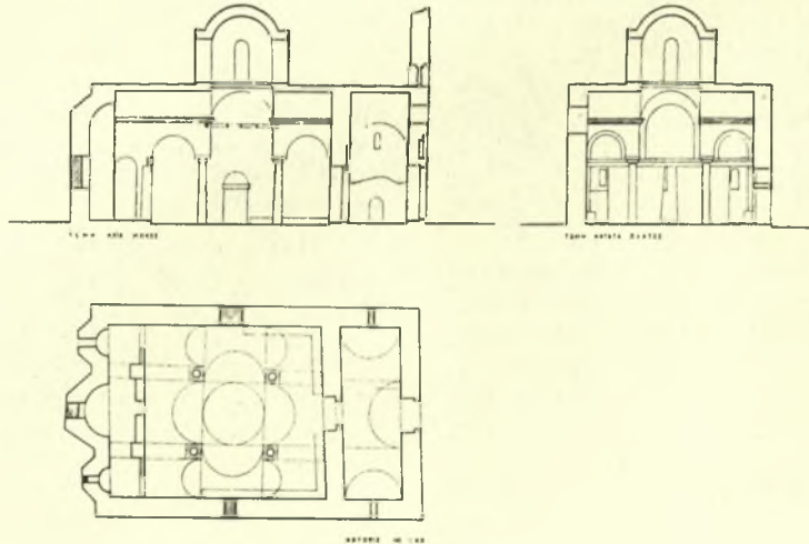
Σχέδ. 1. Ἁγιος Ἰωάννης Κέριας. Κάτοπις καὶ τομαί
