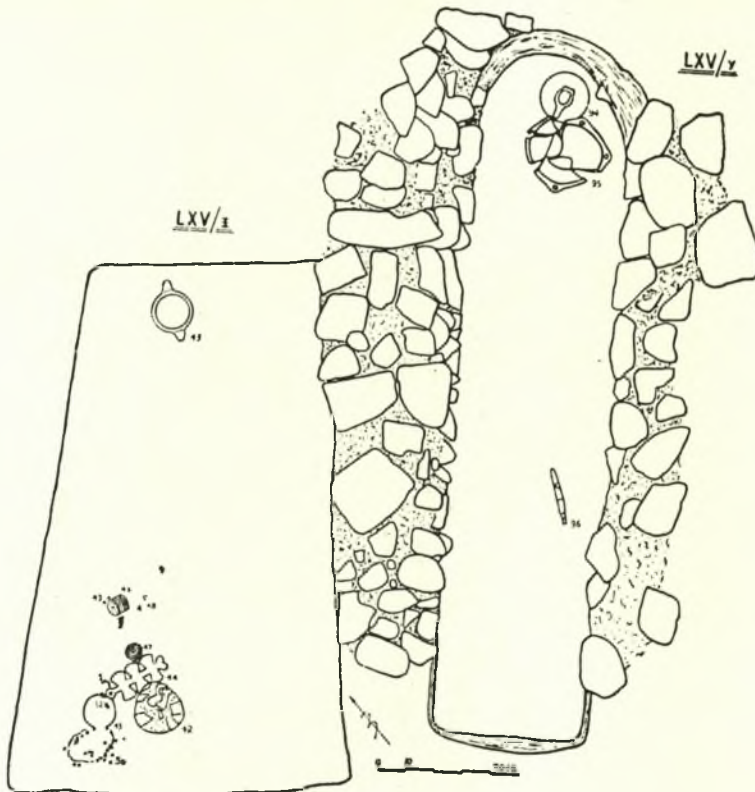
Σχεδ. 54. Τομαί Ξ καὶ Υ τοῦ τύμβου LXV
