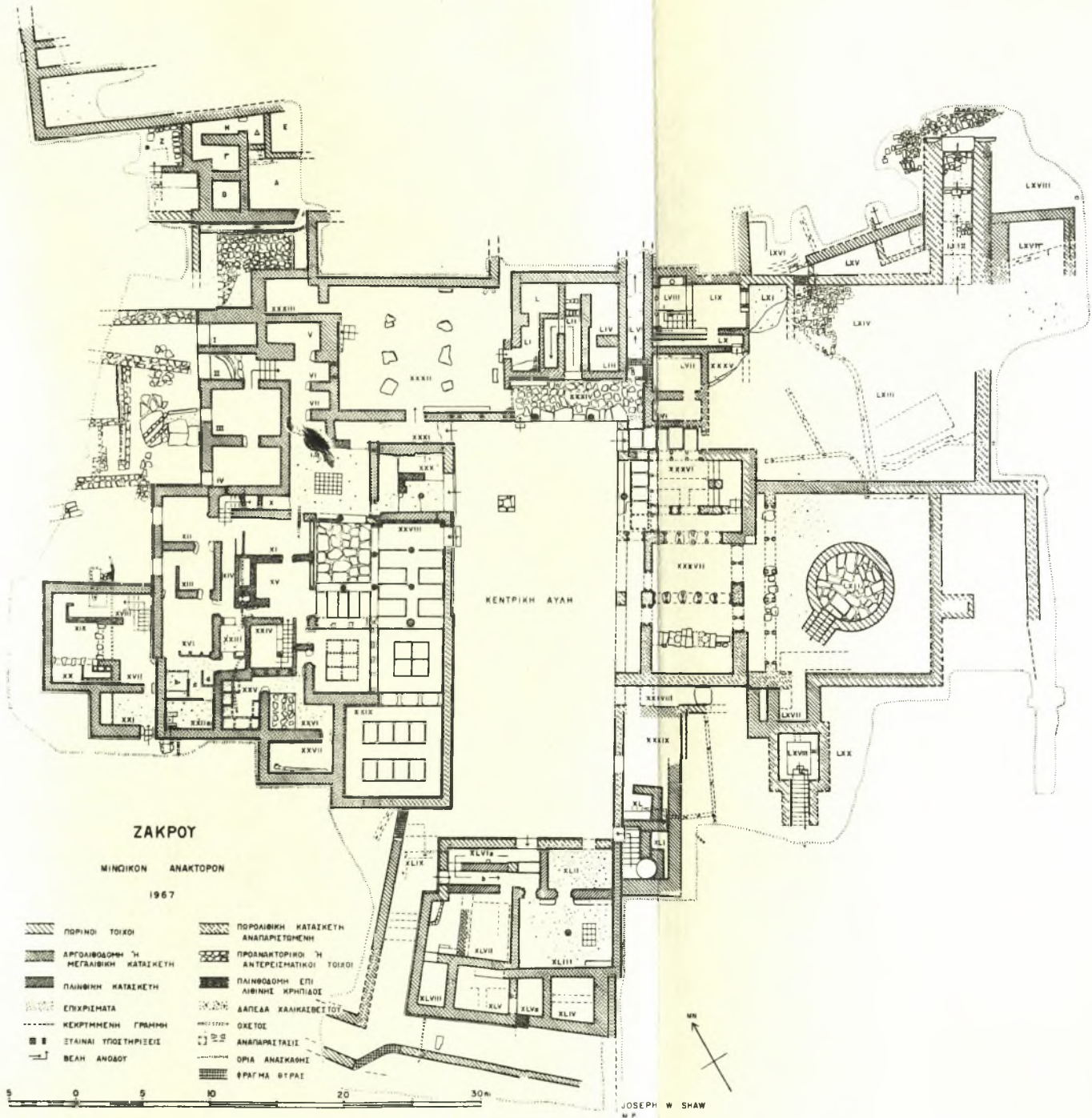
Γενικόν σχέδιον κατόψεως τοῦ ἀνακτόρου Ζάκρου.
