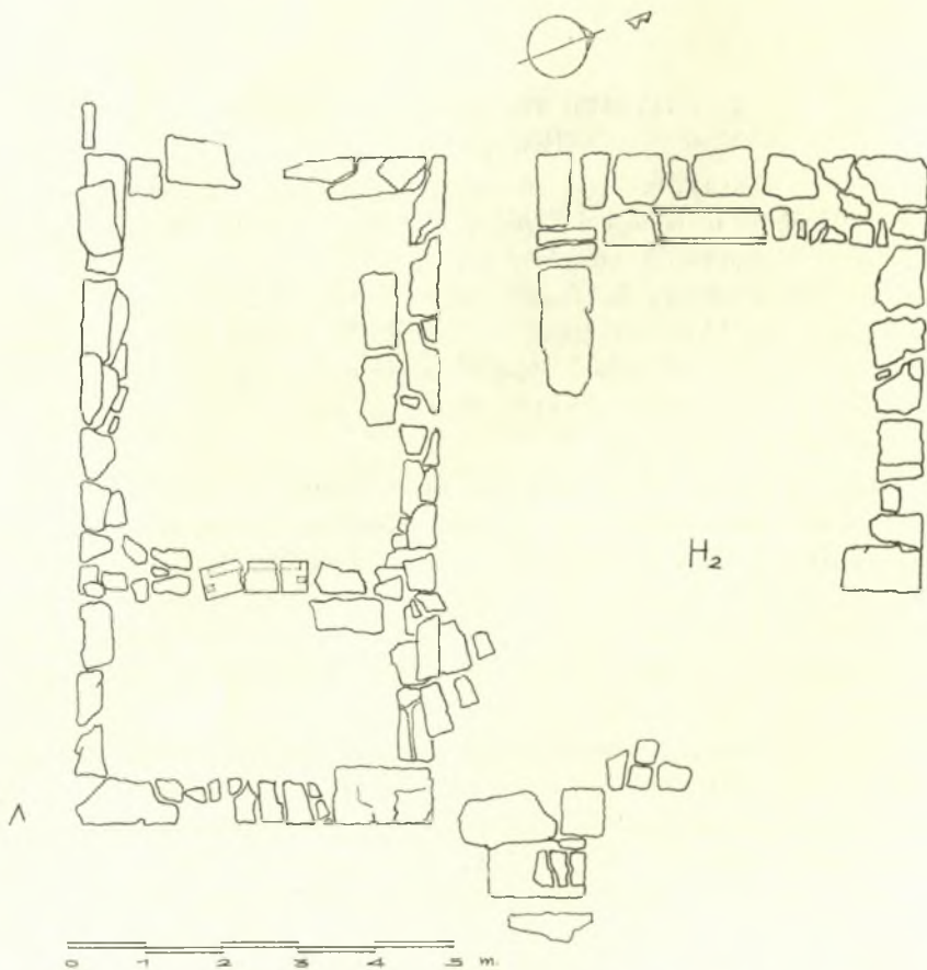
Εἰκ. 1. Κάτοπις ναύσκου Α καὶ ρωμαϊκοῦ κτίσματος Η 2 .
