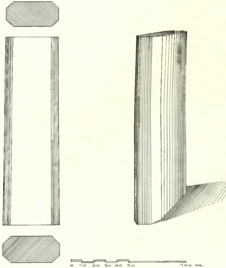
Εἰκ. 3. Τομή, ὄψις καὶ προοπτικὴ μορφή ὀκταπλεύρου στύλου τοῦ ναῦσκου Λ.
