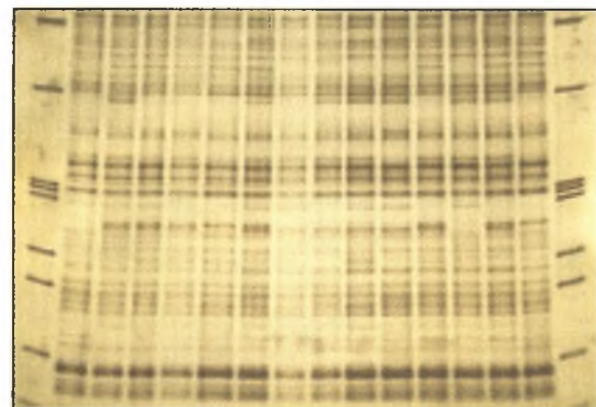
Εικόνα 12. Ανάλυση AFLP για χαρτογράφηση πληθυσμού χειμερινής ελαιοκράμβης.
