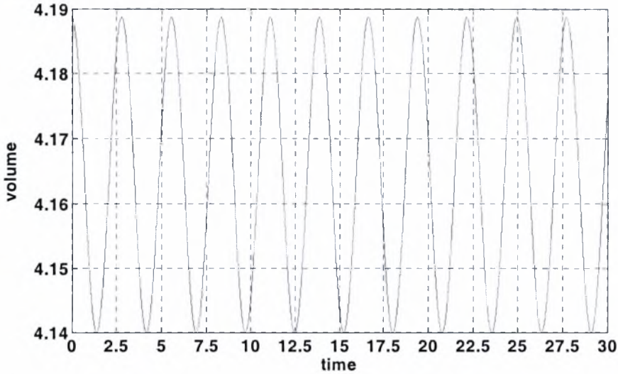
Σχήμα 2. Ο όγκος της μικροφουσαλίδας σε συνάρτηση του χρόνου για γραμμική διαταραχή. Δεδομένα προσομοίωσης: R_{bal}=1.5 \mu\text{m} , G_s=18 \text{ MPa} , \alpha=0.5 , \delta=15 \text{ nm} , \rho_l=998 \text{ kg/m}^3 , P_{st}=1 \text{ atm} , \nu_l=2.4 \text{ MHz} , \varepsilon_{inf}=0.05 , \gamma=1.4 , αριθμός στοιχείων 60.
