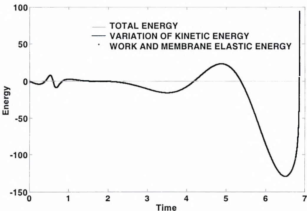
Σχήμα 3. Η συνολική ενέργεια της μικροφουσαλίδας συναρτήσει του χρόνου. Δεδομένα προσομοίωσης: R_{bal}=1.5 \mu\text{m} , G_s=18 \text{ MPa} , \alpha=0.5 , \delta=15 \text{ nm} , \rho_l=998 \text{ kg/m}^3 , P_{st}=1 \text{ atm} , v_f=2.4 \text{ MHz} , \varepsilon_{int}=12 , \gamma=1.4 , αριθμός στοιχείων 100.
