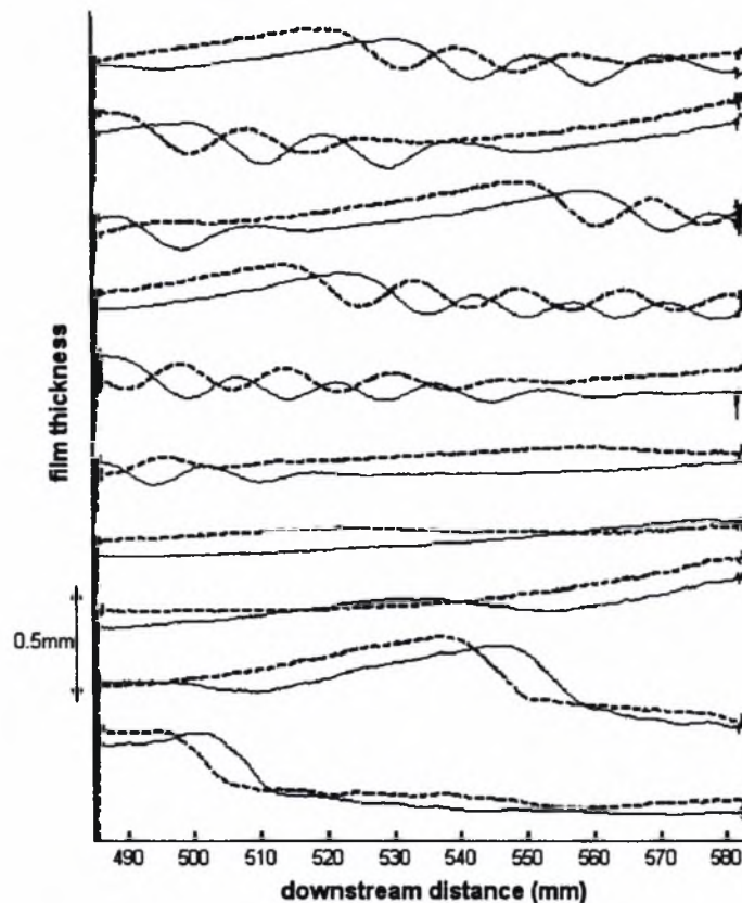
Σχήμα 4.8: Προφίλ 2 διαδοχικών κύκλων της διαταραχής σε συνθήκες ροής Re=32 , \varphi=3.4^\circ , f=0.26 Hz (ο ένας έχει μετακινηθεί ελαφρώς οριζόντια για την καλύτερη παρουσίαση). Παρατηρείται η ίδια χώρο – χρονική εξέλιξη της ροής και της δημιουργίας των παρασιτικών καμπυλών.
