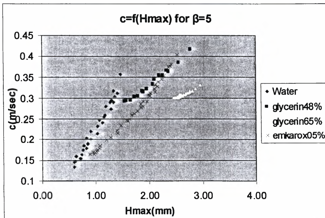
Σχήμα 4.1: c = f(H_{max}) για ρευστά με διαφορετικό ιξώδες.
