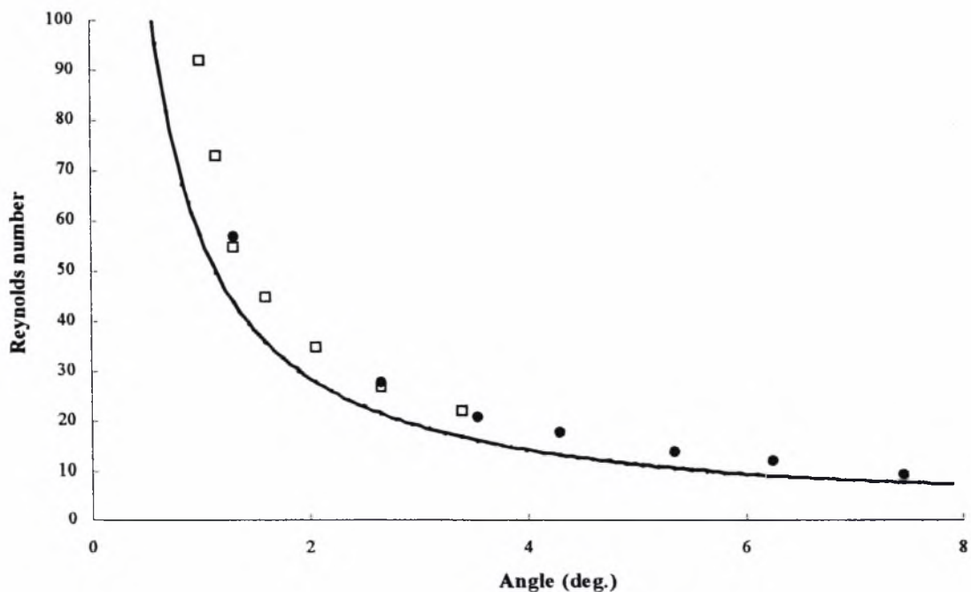
Σχήμα 2.2: Ο κρίσιμος αριθμός Re , για την πρωταρχική αστάθεια του υμένα, μετρούμενος ως συνάρτηση της γωνίας κλίσης, στην περίπτωση χρήσης ορθογώνιου τοιχώματος. (□) Ka=3365 , (●) Ka=1102 , (—) Re=5/6 \cot \theta .
