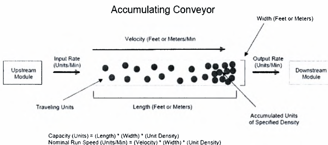
Σχήμα 3-4: Ιμάντας Συγκέντρωσης
