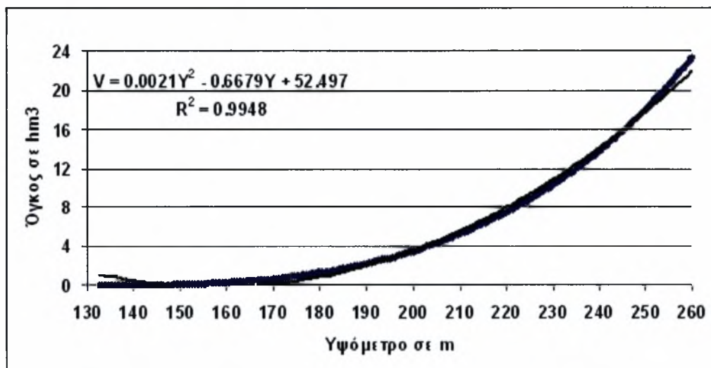
Σχήμα 6.2.4 Καμπύλη Όγκου – Υψόμετρου Ταμιευτήρα Κλινοβός
