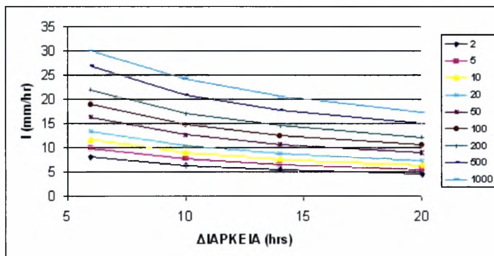
Σχήμα 5.5.13. Όμβριες καμπύλες Έντασης – Διάρκειας – Συχνότητας βροχόπτωσης, για διάφορες περιόδους επαναφοράς, του σταθμού της Σκοπιάς.
