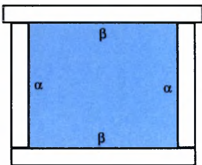
Εικ. 18: Υπολογισμός υδραυλικής ακτίνας για ημιγεμή και πλήρη αγωγό ορθγωνικής διατομής
