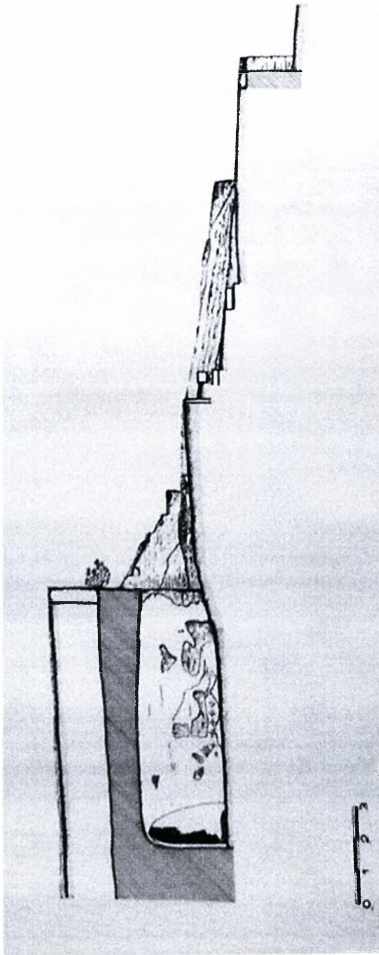
Εικ 54: Πλευρική τομή της κρήνης της Κύθνου στον άξονα ΑΑ της εικ. 45 (σχ. Α. Γούναρης — πηγή: Α. Μαζαράκης Αινιάν, «Επιφανειακές αρχαιολογικές έρευνες στην Κύθνο», ΠΑΕ 1995, σ. 192, εικ. 40)
