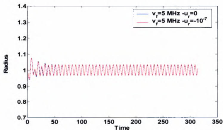
Σχήμα 4.67: Η ακτίνα της μικροφουσαλίδας ως συνάρτηση του χρόνου με και χωρίς παραμένουσες τάσεις στη μεμβράνη εκτός συντονισμού. Δεδομένα προσομοίωσης: \gamma=1.4 , P_{inf}=101325 Pa, \rho_l=998 , kg/m 3 , s=0.045 kg/s 2 , \mu_l=0.001 kgm -1 s -1 , C_l=1500 m/s, \mu_s=0.6 kgm -1 s -1 , G_s=35 MPa, r=3*10^{-6} m, \delta=15*10^{-9} m, \epsilon_{inf}=0.05, b=0
