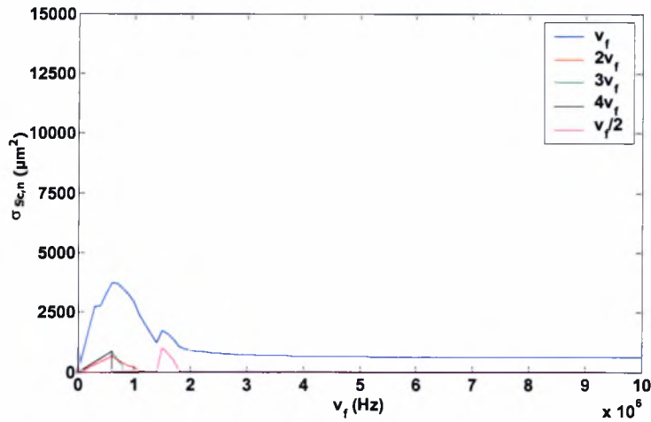
Σχήμα 4.48: Το \sigma_{sc,n} ως συνάρτηση της εξωτερικής συχνότητας για r=7*10^{-6} m. Δεδομένα προσομοίωσης: \gamma=1.4 , P_{inf}=101325 Pa, \rho_l=998 kg/m 3 , s=0.045 kg/s 2 , \mu_l=0.001 kgm -1 s -1 , C_l=1500 m/s, G_s=35 MPa, \mu_s=0.6 kgm -1 s -1 , \delta=15*10^{-9} m, \epsilon_{inf}=2.05 , u_r(t=0)|_{r=1} = u_r(t=0)|_{r=R_{bol}} = 0 , b=0
