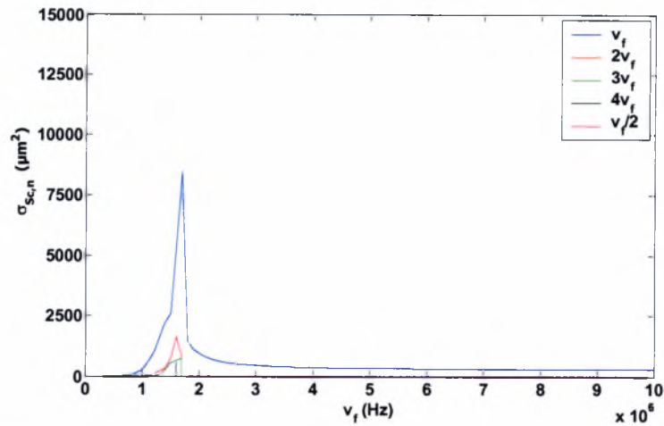
Σχήμα 4.50: Το \sigma_{sc,n} ως συνάρτηση της εξωτερικής συχνότητας για r=5 \cdot 10^{-6} m. Δεδομένα προσομοίωσης: \gamma=1.4 , P_{inf}=101325 Pa, \rho_l=998 kg/m 3 , s=0.045 kg/s 2 , \mu_l=0.001 kgm -1 s -1 , C_l=1500 m/s, G_s=35 MPa, \mu_s=0.6 kgm -1 s -1 , \delta=15 \cdot 10^{-9} m, \epsilon_{inf}=2.05 , u_r(t=0)|_{r=1} = u_r(t=0)|_{r=R_{bal}} = 0 , c=1
