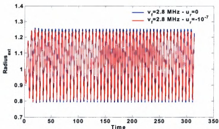
Σχήμα 4-78: Η εξωτερική ακτίνα της μικροφουσαλίδας ως συνάρτηση του χρόνου με και χωρίς παραμένουσες τάσεις στη μεμβράνη σε συντονισμό. Δεδομένα προσομοίωσης: \gamma=1.4 , P_{inf}=101325 Pa, \rho_l=998 kg/m 3 , s_1=0.04 kg/s 2 , s_2=0.005 kg/s 2 , \mu_l=0.001 kgm -1 s -1 , C_l=1500 m/s, \mu_s=0.6 kgm -1 s -1 , G_s=35 MPa, \alpha=3 \cdot 10^{-6} m, \delta=15 \cdot 10^{-9} m, \epsilon_{inf}=0.05 .
