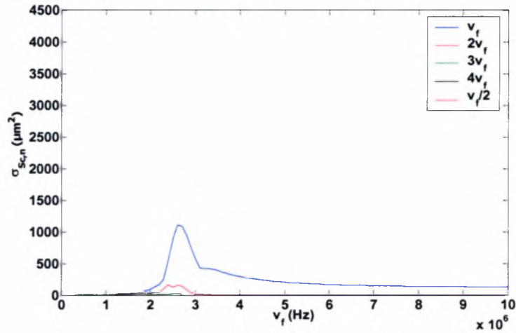
Σχήμα 4.80: Contrast Agent (μοντέλο Mooney-Rivlin). Δεδομένα προσομοίωσης: \gamma=1.4 , P_{inf}=101325 Pa, \rho_l=998 kg/m 3 , s=0.045 kg/s 2 , \mu_l=0.001 kgm -1 s -1 , C_l=1500 m/s, \alpha=3 \cdot 10^{-6} m, G_s=35 MPa, \mu_s=0.6 kgm -1 s -1 , \delta=15 \cdot 10^{-9} m, \epsilon_{inf}=1.0 , u_r(t=0)|_{r=1} = u_r(t=0)|_{r=R_{bal}} = 0 , b=0
