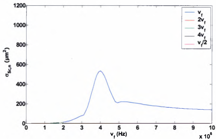
Σχήμα 4.39: Το \sigma_{sc,n} ως συνάρτηση της εξωτερικής συχνότητας για \delta=35*10^{-9} . Δεδομένα προσομοίωσης: \gamma=1.4 , P_{inf}=101325 Pa, \rho_l=998 kg/m 3 , s=0.045 kg/s 2 , \mu_l=0.001 kgm -1 s -1 , C_l=1500 m/s, \mu_s=0.6 kgm -1 s -1 , G_s=35 MPa, r=3*10^{-6} m, \epsilon_{inf}=2.05 , u_r(t=0)|_{r=l} = u_r(t=0)|_{r=R_{bal}} = 0 , c=1
