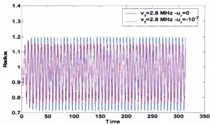
Σχήμα 4.73: Η ακτίνα της μικροφουσαλίδας ως συνάρτηση του χρόνου με και χωρίς παραμένουσες τάσεις στη μεμβράνη σε συντονισμό. Δεδομένα προσομοίωσης: \gamma=1.4 , P_{inf}=101325 Pa, \rho_l=998 kg/m 3 , s=0.045 kg/s 2 , \mu_l=0.001 kgm -1 s -1 , C_l=1500 m/s, \mu_s=0.6 kgm -1 s -1 , G_s=35 MPa, r=3 \cdot 10^{-6} m, \delta=15 \cdot 10^{-9} m, \epsilon_{inf}=0.05 , c=1 .
