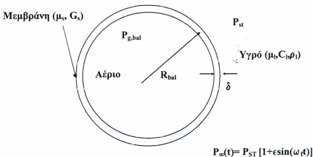
Σχήμα 2-1: Γεωμετρικά χαρακτηριστικά φουσαλίδας σε κατάσταση ισορροπίας
