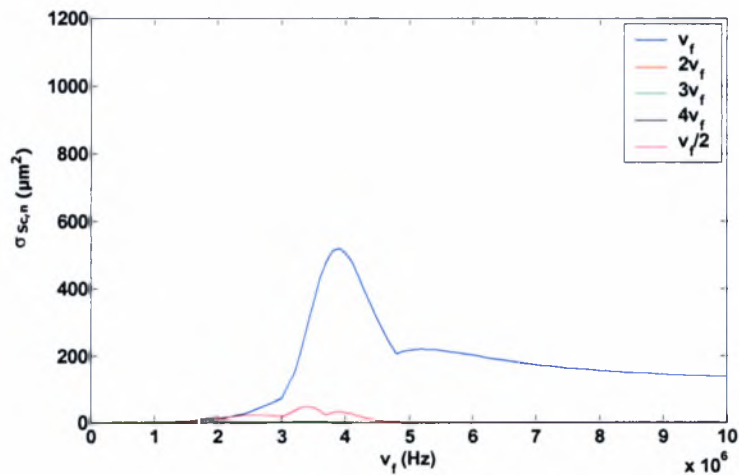
Σχήμα 4.35: Το \sigma_{Sc,n} ως συνάρτηση της εξωτερικής συχνότητας για \delta=35 \cdot 10^{-9} . Δεδομένα προσομοίωσης: \gamma=1.4 , P_{inf}=101325 Pa, \rho_l=998 kg/m 3 , s=0.045 kg/s 2 , \mu_l=0.001 kgm -1 s -1 , C_l=1500 m/s, \mu_s=0.6 kgm -1 s -1 , G_s=35 MPa, r=3 \cdot 10^{-6} m, \epsilon_{inf}=2.05 , u_r(t=0)|_{r=1} = u_r(t=0)|_{r=R_{bol}} = 0 , b=0
