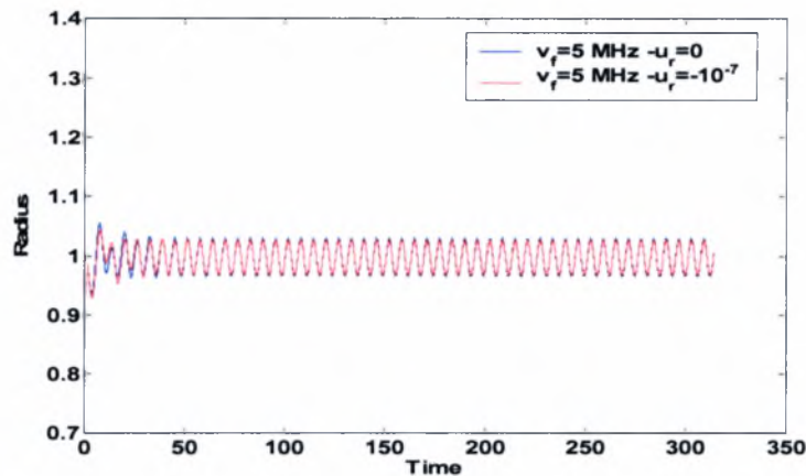
Σχήμα 4.72: Η ακτίνα της μικροφουσαλίδας ως συνάρτηση του χρόνου με και χωρίς παραμένουσες τάσεις στη μεμβράνη εκτός συντονισμού. Δεδομένα προσομοίωσης: \gamma=1.4 , P_{inf}=101325 Pa, \rho_l=998 , kg/m 3 , s=0.045 kg/s 2 , \mu_l=0.001 kgm -1 s -1 , C_l=1500 m/s, \mu_s=0.6 kgm -1 s -1 , G_s=35 MPa, r=3 \cdot 10^{-6} m, \delta=15 \cdot 10^{-9} m, \epsilon_{inf}=0.05 , b=0 .
