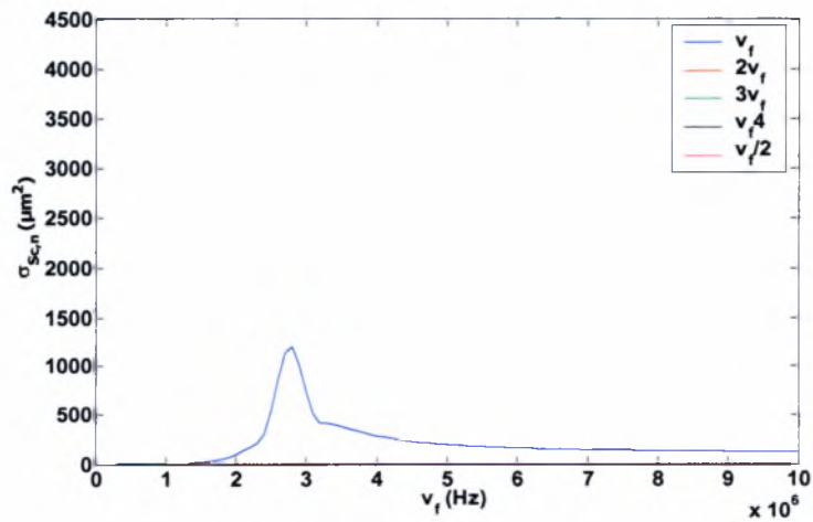
Σχήμα 4.81: Contrast Agent (μοντέλο Skalak). Δεδομένα προσομοίωσης: \gamma=1.4 , P_{inf}=101325 Pa, \rho_l=998 kg/m 3 , s=0.045 kg/s 2 , \mu_l=0.001 kgm -1 s -1 , C_l=1500 m/s, \alpha=3 \cdot 10^{-6} m, G_s=35 MPa, \mu_s=0.6 kgm -1 s -1 , \delta=15 \cdot 10^{-9} m, \epsilon_{inf}=1.0 , u_r(t=0)|_{r=1} = u_r(t=0)|_{r=R_{bal}} = 0 , c=1
