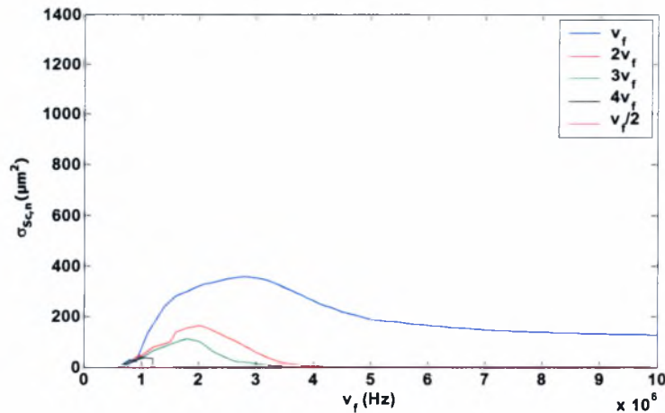
Σχήμα 4.3: Το \sigma_{sc,n} ως συνάρτηση της εξωτερικής συχνότητας για \varepsilon_{inf}=4.05 . Δεδομένα προσομοίωσης: \gamma=1.4 , P_{inf}=101325 Pa, \rho_l=998 kg/m 3 , s=0.045 kg/s 2 , \mu_l=0.001 kgm -1 s -1 , C_l=1500 m/s, \mu_s=0.6 kgm -1 s -1 , G_s=35 MPa, r=3 \cdot 10^{-6} m, \delta=15 \cdot 10^{-9} m, u_r(t=0)|_{r=1} = u_r(t=0)|_{r=R_{bal}} = 0 , b=0
