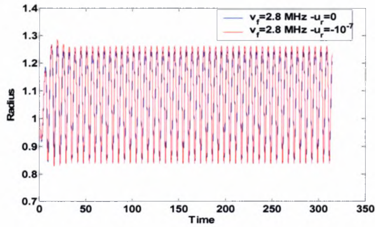
Σχήμα 4.68: Η ακτίνα της μικροφουσαλίδας ως συνάρτηση του χρόνου με και χωρίς παραμένουσες τάσεις στη μεμβράνη σε συντονισμό. Δεδομένα προσομοίωσης: \gamma=1.4 , P_{inf}=101325 Pa, \rho_l=998 kg/m 3 , s=0.045 kg/s 2 , \mu_l=0.001 kgm -1 s -1 , C_l=1500 m/s, \mu_s=0.6 kgm -1 s -1 , G_s=35 MPa, r=3 \cdot 10^{-6} m, \delta=15 \cdot 10^{-9} m, \epsilon_{inf}=0.05 , b=0 .
