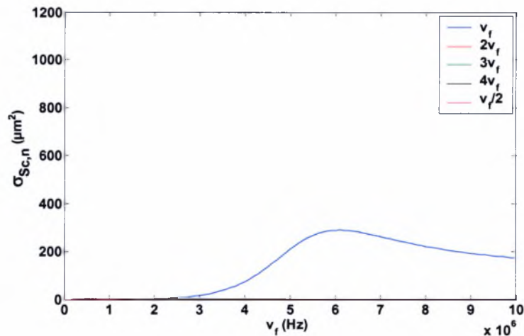
Σχήμα 4.45: Το \sigma_{Sc,n} ως συνάρτηση της εξωτερικής συχνότητας για \delta=75*10^{-9} m. Δεδομένα προσομοίωσης: \gamma=1.4 , P_{inf}=101325 Pa, \rho_l=998 kg/m 3 , s_1=0.04 kg/s 2 , s_2=0.005 kg/s 2 , \mu_l=0.001 kgm -1 s -1 , C_l=1500 m/s, \mu_s=0.6 kgm -1 s -1 , G_s=35 MPa, r=3*10^{-6} m, \epsilon_{inf}=2.05 , u_r(t=0)|_{r=1} = u_r(t=0)|_{r=a_{bal}} = 0
