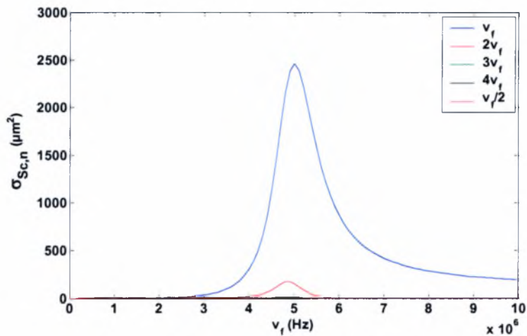
Σχήμα 4.21: Το \sigma_{sc,n} ως συνάρτηση της εξωτερικής συχνότητας για G_s=140 MPa. Δεδομένα προσομοίωσης: \gamma=1.4 , P_{int}=101325 Pa, \rho_l=998 kg/m 3 , s_1=0.04 kg/s 2 , s_2=0.005 kg/s 2 , \mu_l=0.001 kgm -1 s -1 , C_l=1500 m/s, \mu_s=0.6 kgm -1 s -1 , r=3*10^{-6} m, \delta=15*10^{-9} m, \epsilon_{int}=2.05 , u_r(t=0)|_{r=1} = u_r(t=0)|_{r=a_{hol}} = 0
