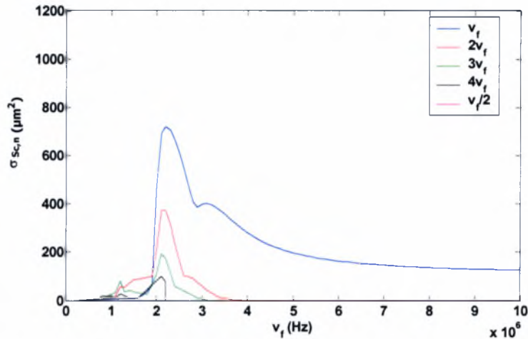
Σχήμα 4.34: Το \sigma_{Sc,n} ως συνάρτηση της εξωτερικής συχνότητας για \delta=15 \cdot 10^{-9} . Δεδομένα προσομοίωσης: \gamma=1.4 , P_{inf}=101325 Pa, \rho_l=998 kg/m 3 , s=0.045 kg/s 2 , \mu_l=0.001 kgm -1 s -1 , C_l=1500 m/s, \mu_s=0.6 kgm -1 s -1 , G_s=35 MPa, r=3 \cdot 10^{-6} m, \epsilon_{inf}=2.05 , u_r(t=0)|_{r=1} = u_r(t=0)|_{r=R_{bol}} = 0 , b=0
