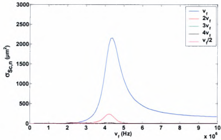
Σχήμα 4.20: Το \sigma_{sc,n} ως συνάρτηση της εξωτερικής συχνότητας για G_s=105 MPa. Δεδομένα προσομοίωσης: \gamma=1.4 , P_{int}=101325 Pa, \rho_l=998 kg/m 3 , s_1=0.04 kg/s 2 , s_2=0.005 kg/s 2 , \mu_l=0.001 kgm -1 s -1 , C_l=1500 m/s, \mu_s=0.6 kgm -1 s -1 , r=3*10^{-6} m, \delta=15*10^{-9} m, \epsilon_{int}=2.05 , u_r(t=0)|_{r=1} = u_r(t=0)|_{r=a_{hol}} = 0
