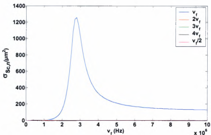
Σχήμα 4.7: Το \sigma_{Sc,n} ως συνάρτηση της εξωτερικής συχνότητας για \epsilon_{inf}=0.05 . Δεδομένα προσομοίωσης: \gamma=1.4 , P_{inf}=101325 Pa, \rho_l=998 kg/m 3 , s_1=0.04 kg/s 2 , s_2=0.005 kg/s 2 , \mu_l=0.001 kgm -1 s -1 , C_l=1500 m/s, \mu_s=0.6 kgm -1 s -1 , G_s=35 MPa, r=3 \cdot 10^{-6} m, \delta=15 \cdot 10^{-9} m, u_r(t=0)|_{r=1} = u_r(t=0)|_{r=a_{bul}} = 0
