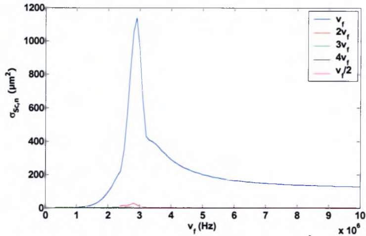
Σχήμα 4.38: Το \sigma_{sc,n} ως συνάρτηση της εξωτερικής συχνότητας για \delta=15*10^{-9} . Δεδομένα προσομοίωσης: \gamma=1.4 , P_{inf}=101325 Pa, \rho_l=998 kg/m 3 , s=0.045 kg/s 2 , \mu_l=0.001 kgm -1 s -1 , C_l=1500 m/s, \mu_s=0.6 kgm -1 s -1 , G_s=35 MPa, r=3*10^{-6} m, \epsilon_{inf}=2.05 , u_r(t=0)|_{r=l} = u_r(t=0)|_{r=R_{bal}} = 0 , c=1
