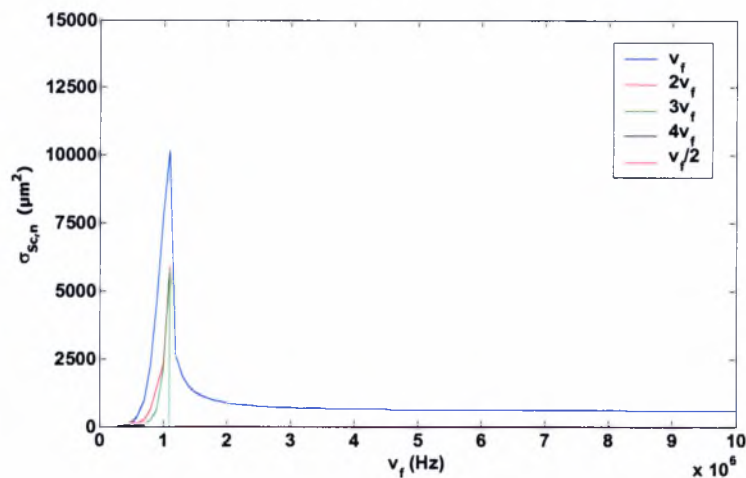
Σχήμα 4.51: Το \sigma_{sc,n} ως συνάρτηση της εξωτερικής συχνότητας για r=7 \cdot 10^{-6} m. Δεδομένα προσομοίωσης: \gamma=1.4 , P_{inf}=101325 Pa, \rho_l=998 kg/m 3 , s=0.045 kg/s 2 , \mu_l=0.001 kgm -1 s -1 , C_l=1500 m/s, G_s=35 MPa, \mu_s=0.6 kgm -1 s -1 , \delta=15 \cdot 10^{-9} m, \epsilon_{inf}=2.05 , u_r(t=0)|_{r=1} = u_r(t=0)|_{r=R_{bal}} = 0 , c=1
