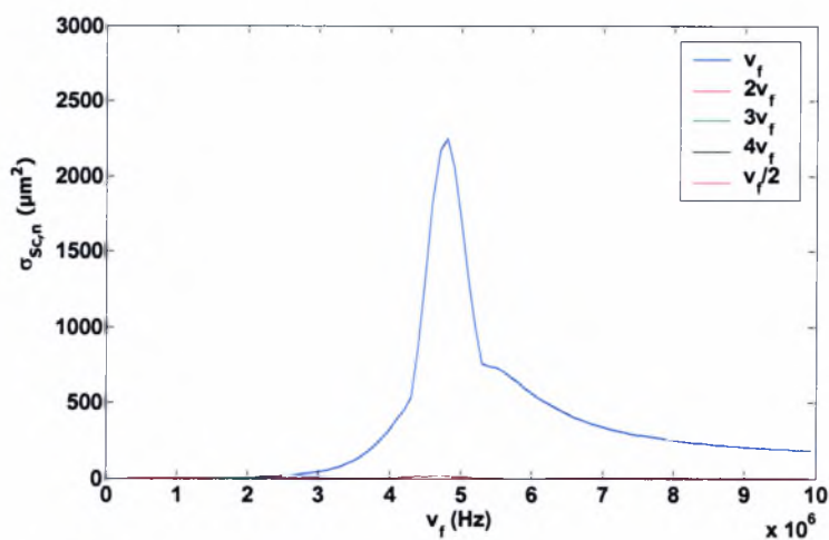
Σχήμα 4.65: Το \sigma_{Sc,n} ως συνάρτηση της εξωτερικής συχνότητας για c=5 . Δεδομένα προσομοίωσης: \gamma=1.4 , P_{inf}=101325 Pa, \rho_l=998 kg/m 3 , s=0.045 kg/s 2 , \mu_l=0.001 kgm -1 s -1 , C_l=1500 m/s, G_s=35 MPa, \mu_s=0.6 kgm -1 s -1 , \delta=15 \cdot 10^{-9} m, \epsilon_{inf}=2.05 , u_r(t=0)|_{r=1} = u_r(t=0)|_{r=R_{hal}} = 0 , r=3 \cdot 10^{-6} m.
