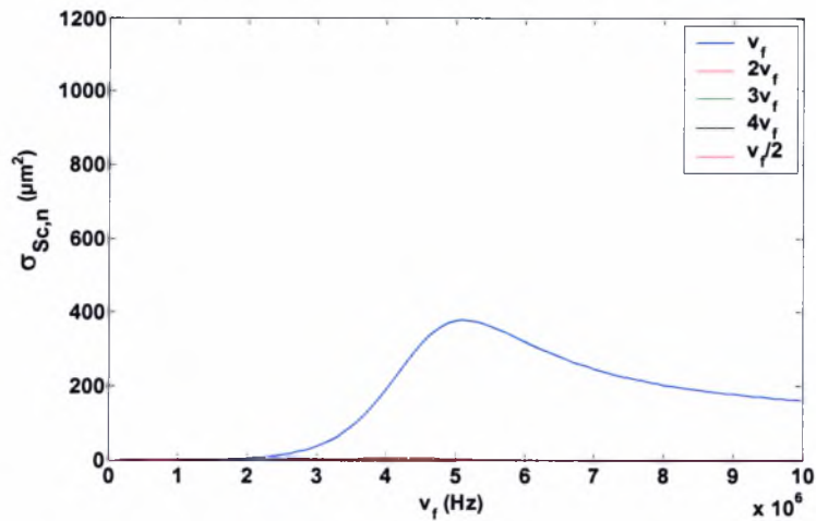
Σχήμα 4.44: Το \sigma_{Sc,n} ως συνάρτηση της εξωτερικής συχνότητας για \delta=55*10^{-9} m. Δεδομένα προσομοίωσης: \gamma=1.4 , P_{inf}=101325 Pa, \rho_l=998 kg/m 3 , s_1=0.04 kg/s 2 , s_2=0.005 kg/s 2 , \mu_l=0.001 kgm -1 s -1 , C_l=1500 m/s, \mu_s=0.6 kgm -1 s -1 , G_s=35 MPa, r=3*10^{-6} m, \epsilon_{inf}=2.05 , u_r(t=0)|_{r=1} = u_r(t=0)|_{r=a_{bal}} = 0
