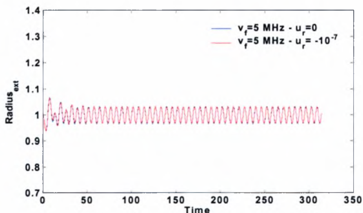
Σχήμα 4-77: Η εξωτερική ακτίνα της μικροφουσαλίδας ως συνάρτηση του χρόνου με και χωρίς παραμένουσες τάσεις στη μεμβράνη εκτός συντονισμού. Δεδομένα προσομοίωσης: \gamma=1.4 , P_{in}=101325 Pa, \rho_l=998 kg/m 3 , s_1=0.04 kg/s 2 , s_2=0.005 kg/s 2 , \mu_l=0.001 kgm -1 s -1 , C_l=1500 m/s, \mu_s=0.6 kgm -1 s -1 , G_s=35 MPa, \alpha=3 \cdot 10^{-6} m, \delta=15 \cdot 10^{-9} m, \epsilon_{in}=0.05 .
