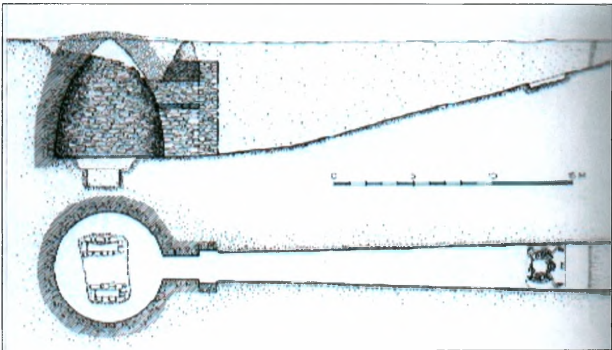
Εικ. 3. Θολωτός τάφος Μαραθώνα : Κάτοψη και τομή.
