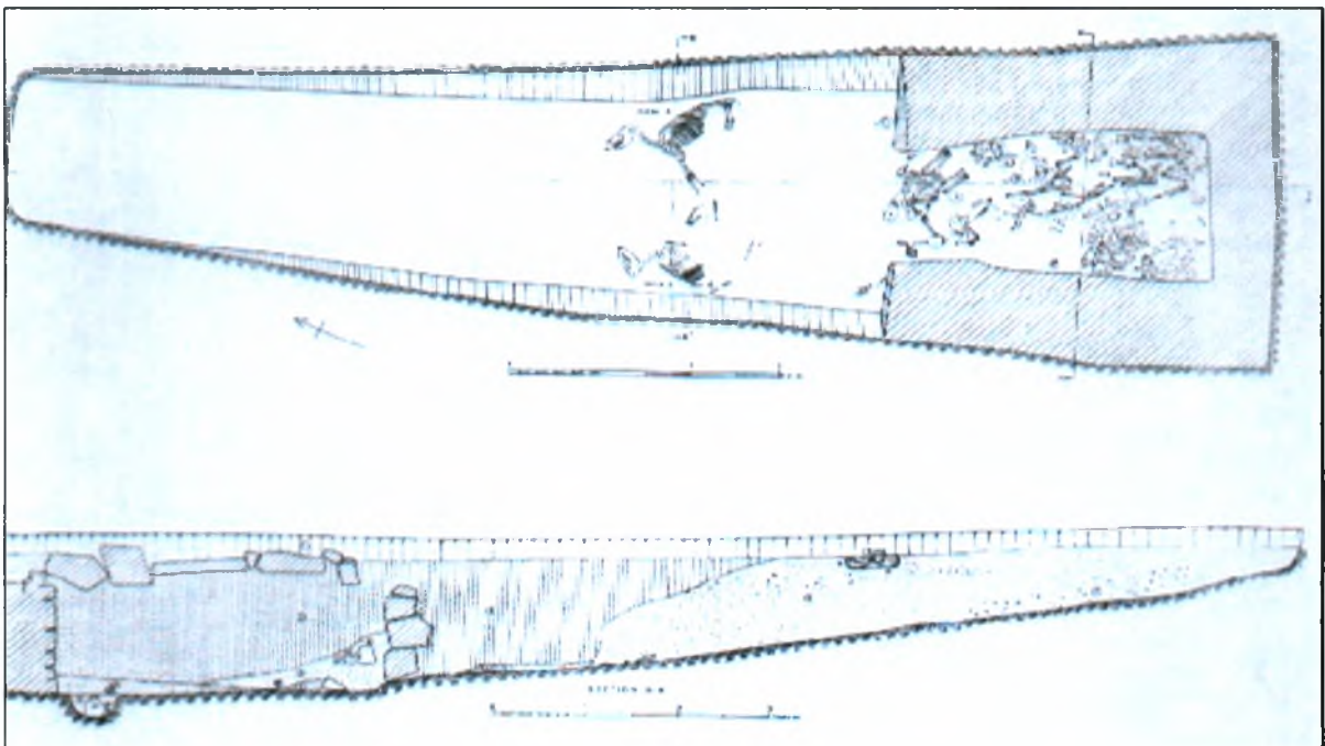
Εικ. 64. Τάφος 31. Επάνω: Σχέδιο με τα ευρήματα του δρόμου και του θαλάμου κατά χώραν. Κάτω: Τομές Α-Α' από βορρά προς νότο.
