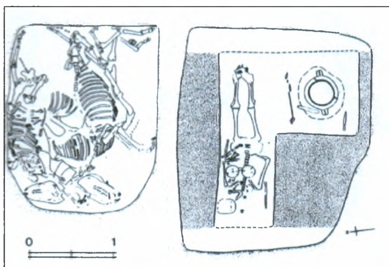
Εικ. 28. Λευκαντί. Τούμπα. Κάτοψη τάφων στο εσωτερικό του αφιδωτού κτιρίου.
