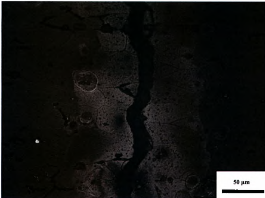
Σχήμα 4.99: Διακρυσταλλική ρωγή στο δοκίμιο 12a ( \sigma_{max} = 150 , N_f = 115.779 ).
