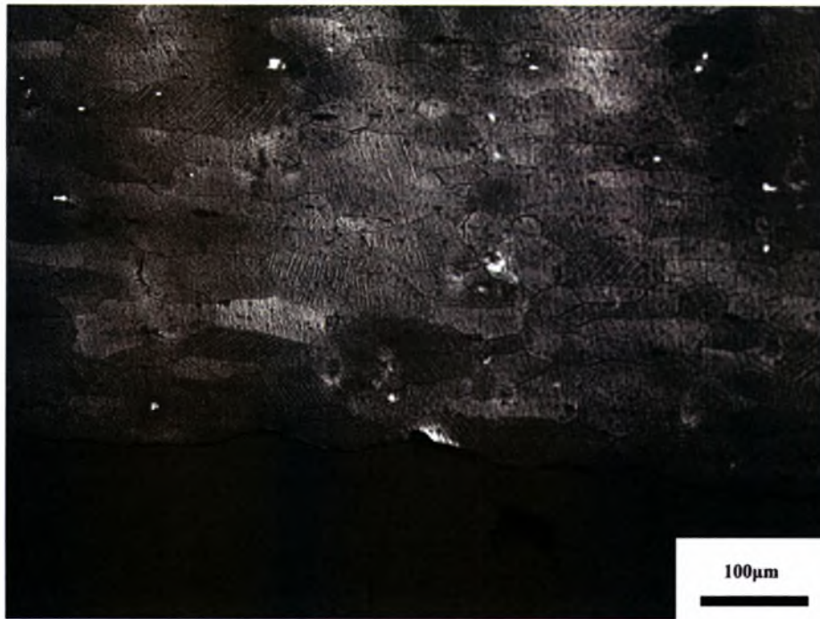
Σχήμα 4.89: Έντονη διάβρωση μακριά από τη ρίζα της συγκόλληση στο δοκίμιο 10a ( \sigma_{\max} = 100 , N_f = 360.266 ).
