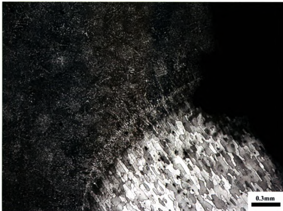
Σχήμα 4.32: Έντονη τρηματική διάβρωση στη συγκόλληση στο δοκίμιο 3a ( \sigma_{\max} = 75 , N_f = 857.628 ).
