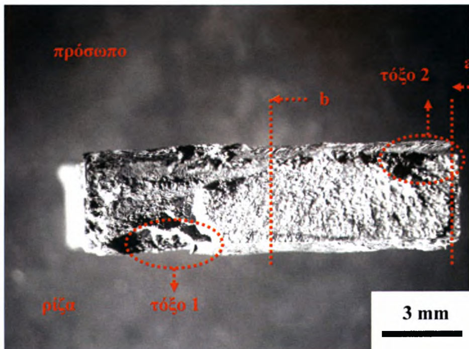
Σχήμα 4.28: Επιφάνεια θραύσης του δοκιμίου 3 ( \sigma_{\max} = 75 , N_f = 857.628 ).
