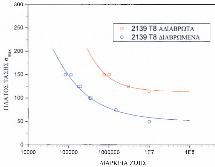
Διάγραμμα 4.51: Καμπύλες Whoeler του κράματος 2139-T8.
