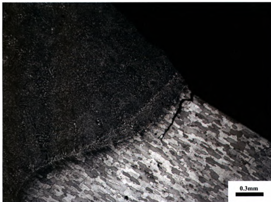
Σχήμα 4.20: Δευτερεύουσα ρωγή κόπωσης στη ZMT στο δοκίμιο 8a ( \sigma_{max} = 150 , N_f = 1.025.613,50 ).
