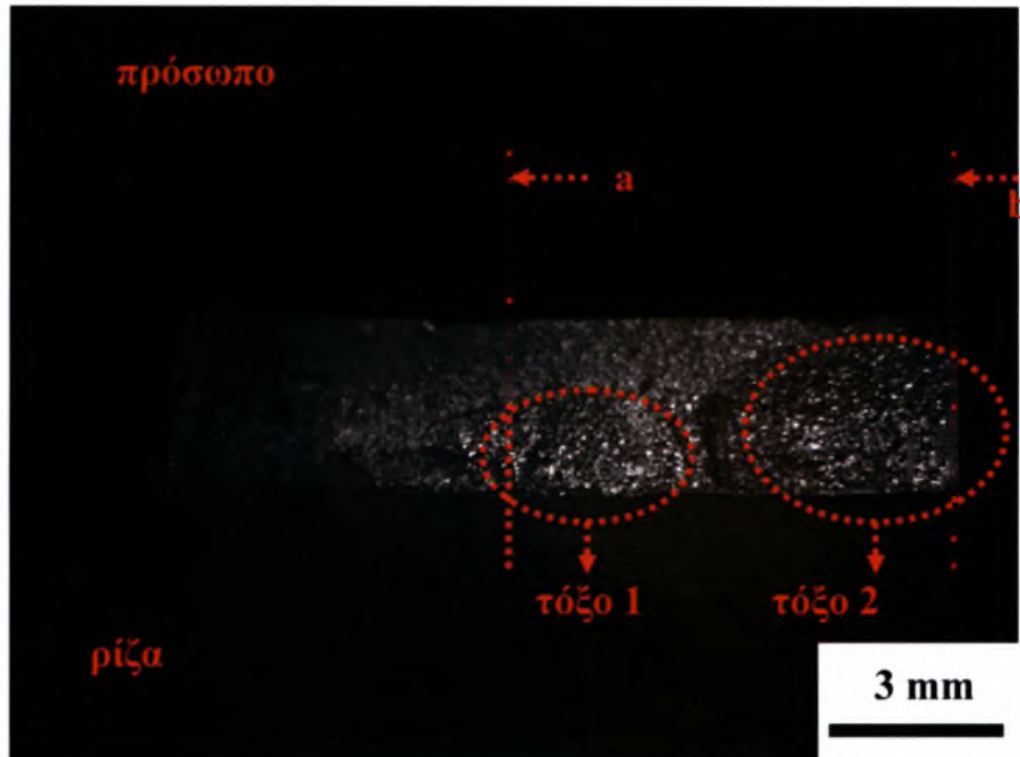
Σχήμα 4.91: Επιφάνεια θραύσης του δοκιμίου 12 ( \sigma_{max} = 150 , N_f = 115.779 ).
