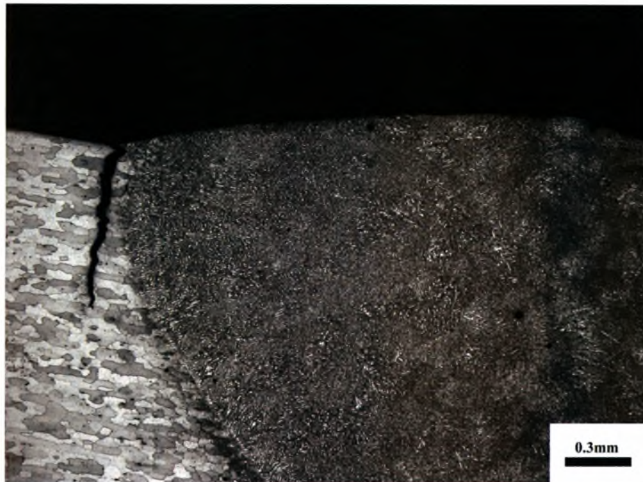
Σχήμα 4.21: Δευτερεύουσα ρωγή κόπωσης στη ZMT στο δοκίμιο 8b ( \sigma_{max} = 150 , N_f = 1.025.613,50 ).
