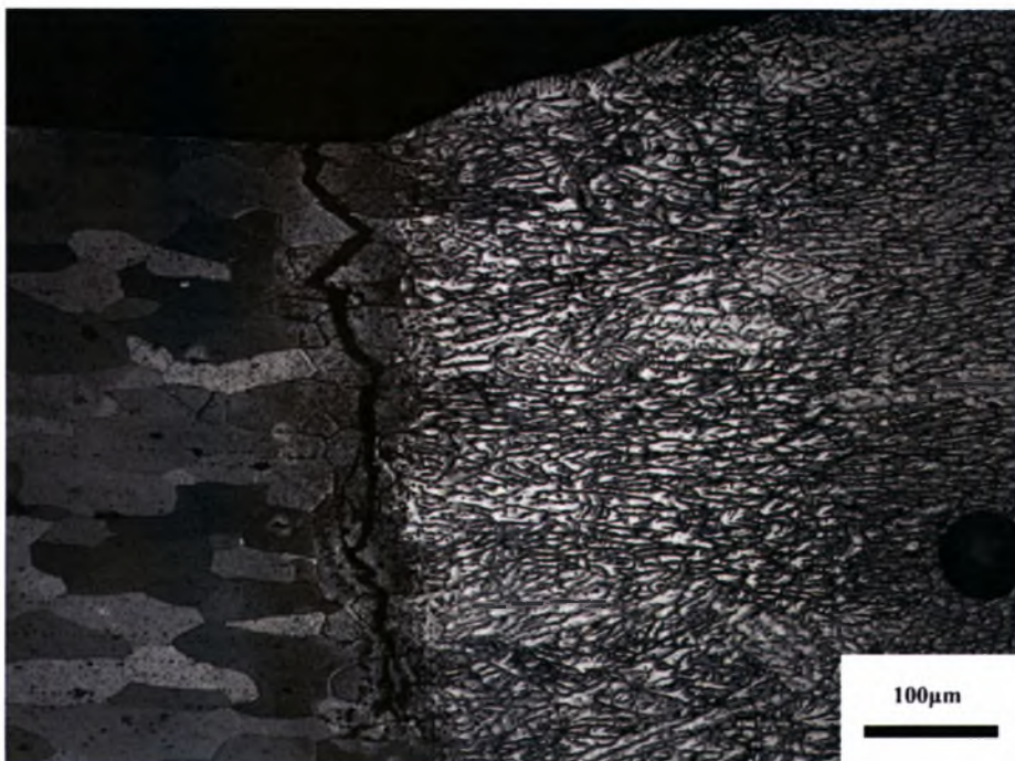
Σχήμα 4.58: Δευτερεύουσα ρωγή κόπωσης στη ZMT στο δοκίμιο 15b ( \sigma_{\max} = 150 , N_f = 1.020.939,50 ).
