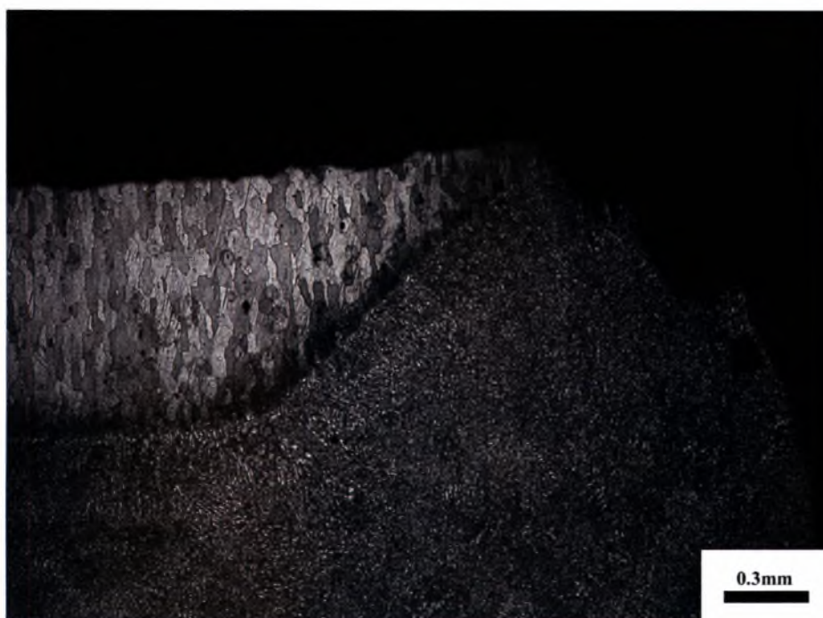
Σχήμα 4.38: Εκκίνηση ρωγμής κόπωσης στο πρόσωπο της συγκόλλησης και διάδοσή της στο μέταλλο συγκόλλησης στο δοκίμιο 4a ( \sigma_{\max} = 100 , N_f = 344.410 ).
