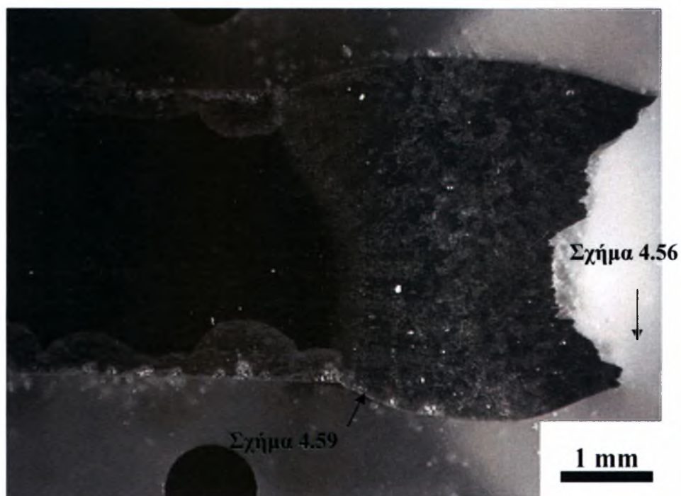
Σχήμα 4.54: Μακρογραφία δοκίμιου 15a ( \sigma_{max} = 150 , N_f = 1.020.939,50 ).
