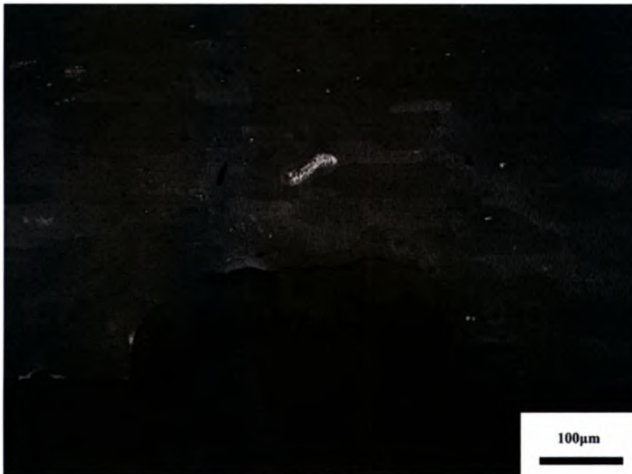
Σχήμα 4.90: Έντονη διάβρωση μακριά από τη ρίζα της συγκόλληση στο δοκίμιο 10b ( \sigma_{\max} = 100 , N_f = 360.266 ).
