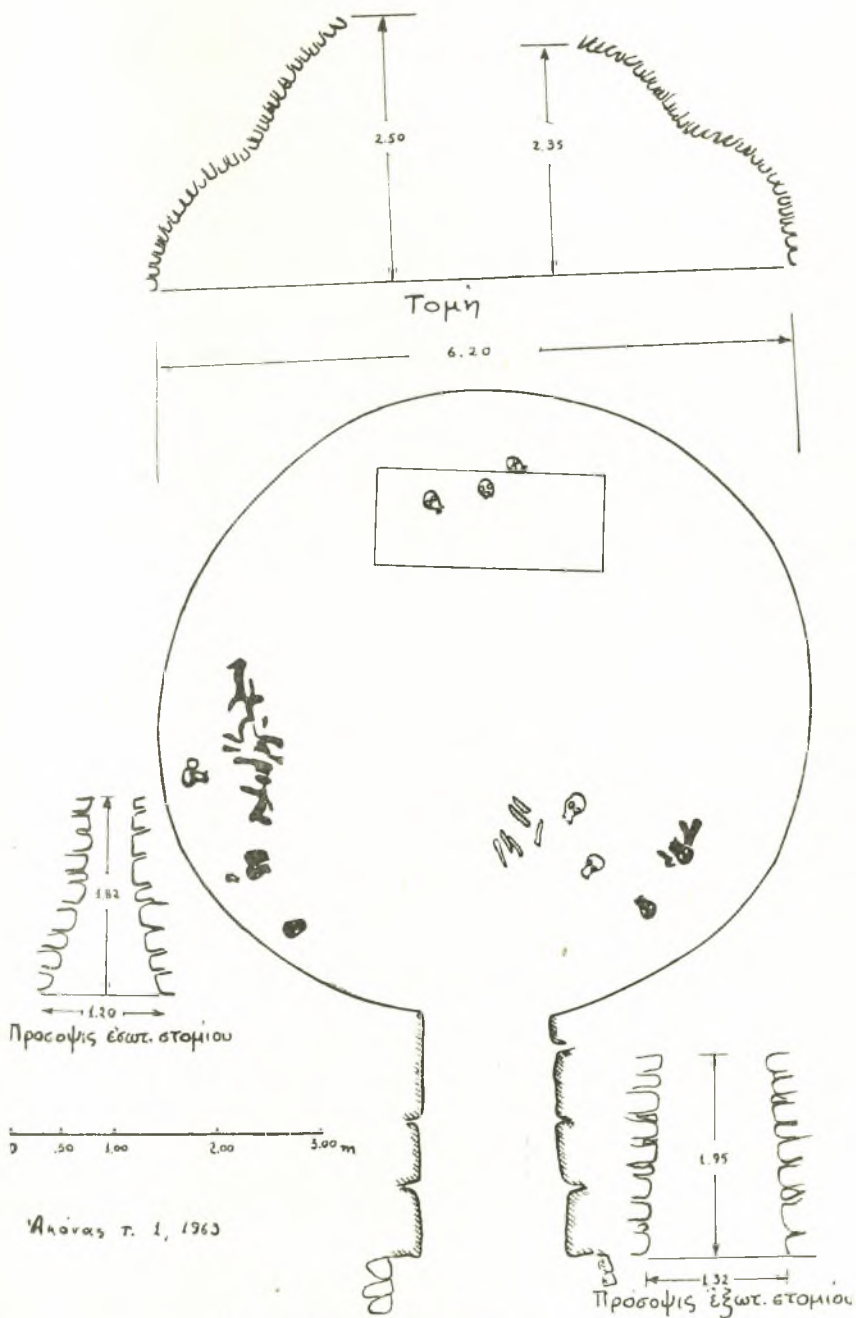
Εικ. 1. Άχνας τ. 1, κάτοψis και τομαί.
