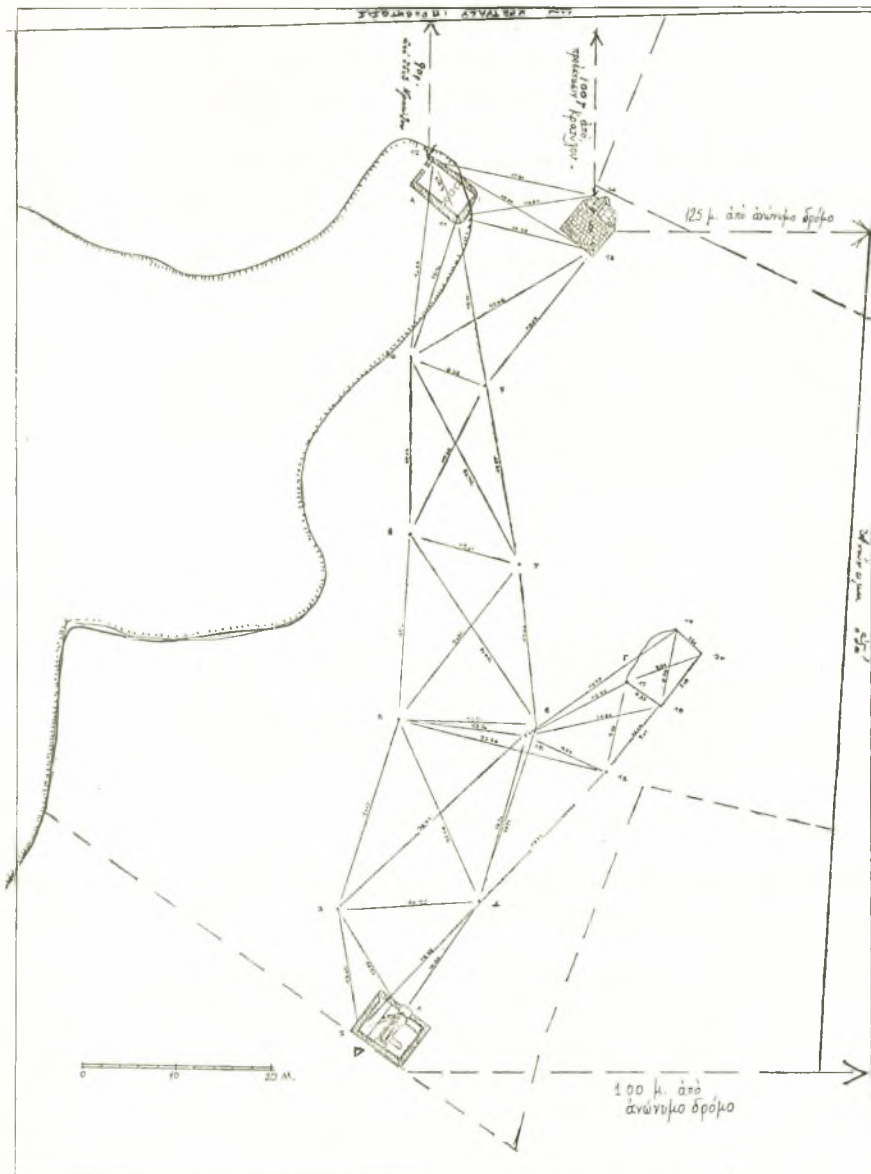
Εικ. 7. Τοπογραφικόν σχέδιον «Χωματερής» Μαυρίκη.
