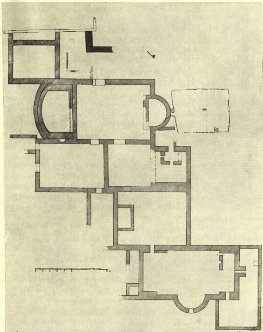
Εἰκ. 1. Γενικὴ κάτοψις τοῦ ἐν Κερκύρα ρωμαϊκοῦ βαλανείου. Ἄνω δεξιὰ ὁ νεοανασκαφίς χώρος ΑΒ.
