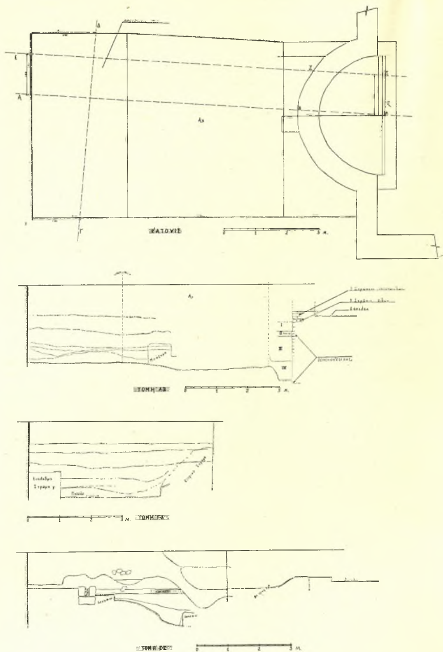
Εικ. 2. Κάτοψις και τομαί του νεοανασκαφέντος χώρου ΑΒ του ἐν Κερκύρα ρωμαϊκοῦ βαλανείου.
