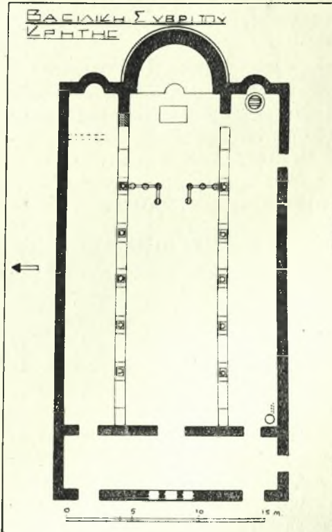
Εἰκ. 1. — Κάτοψις τῆς βυζαντινῆς βασιλικῆς Συβριτοῦ.
