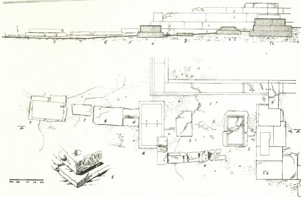
Εικ. 67. Κάτοψις και τομή βάθρων πρό της ΝΔ. πλευράς της Ίερας Οικίας.
