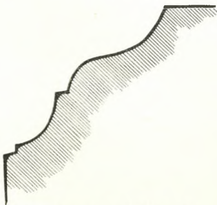
Εἰκ. 69. Τομὴ τῶν κυματίων τοῦ βάθρου 2. Σμίκρονσις 1/3.
