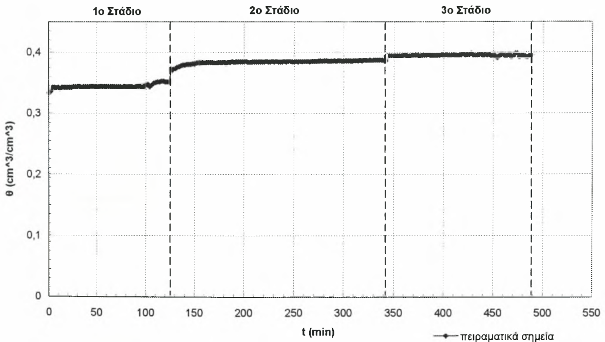
Σχήμα 3.19 Εδαφική υγρασία σε συνάρτηση με το χρόνο, κατά την 2^{\text{η}} διύγρανση
