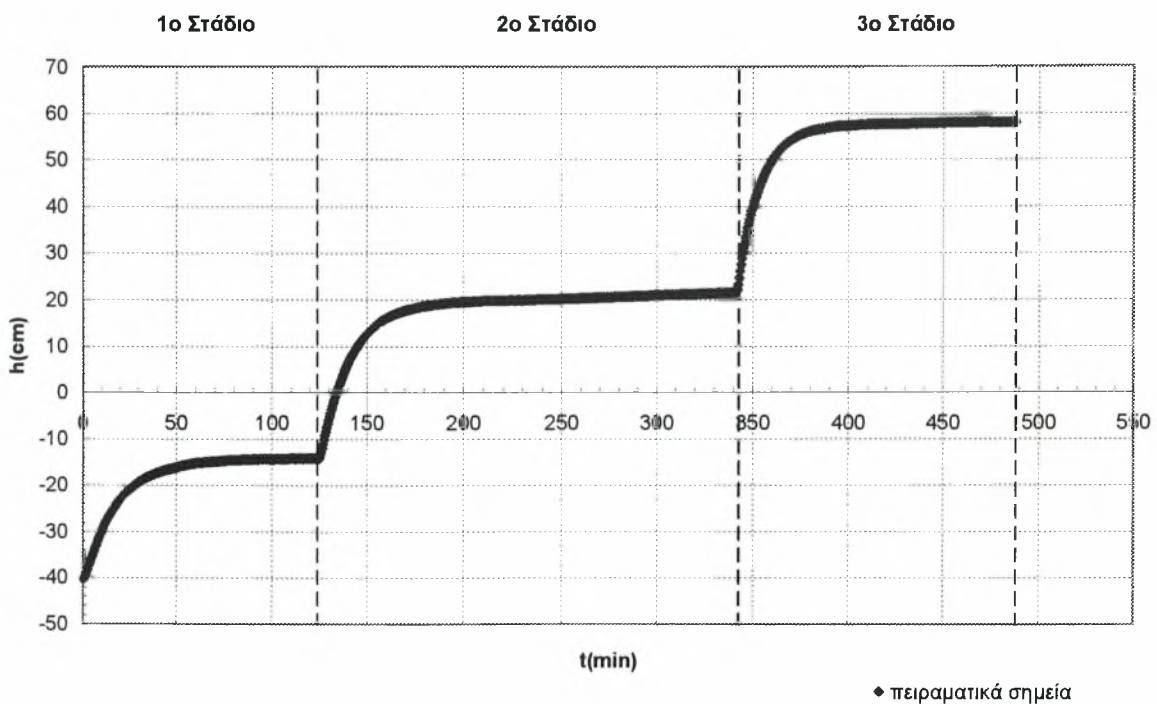
Σχήμα 3.20 Πίεση σε συνάρτηση με το χρόνο, κατά την 2 η διύγρανση
