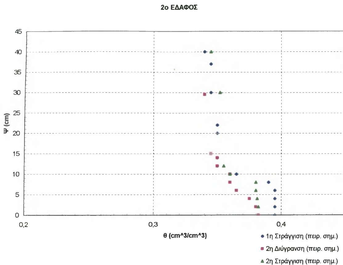
Σχήμα 3.23 Χαρακτηριστικές καμπύλες του εδαφικού δείγματος, για την 1 η στράγγιση, τη 2 η διύγρανση και τη 2 η στράγγιση
