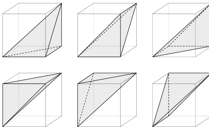
Σχήμα 9.4: Παράδειγμα διαμερισμού κυρτού πολυέδρου (κύβου) σε τετράεδρα.
