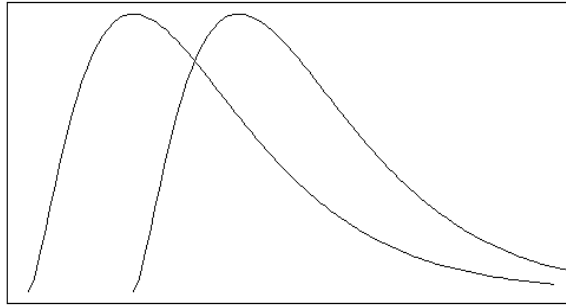
Σχήμα 2.38: Όμοιες κατανομές με διαφορετικές διάμεσους.
