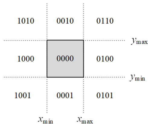
Σχήμα 2.25: Οι κωδικοί περιοχών του αλγορίθμου Skala 2005
