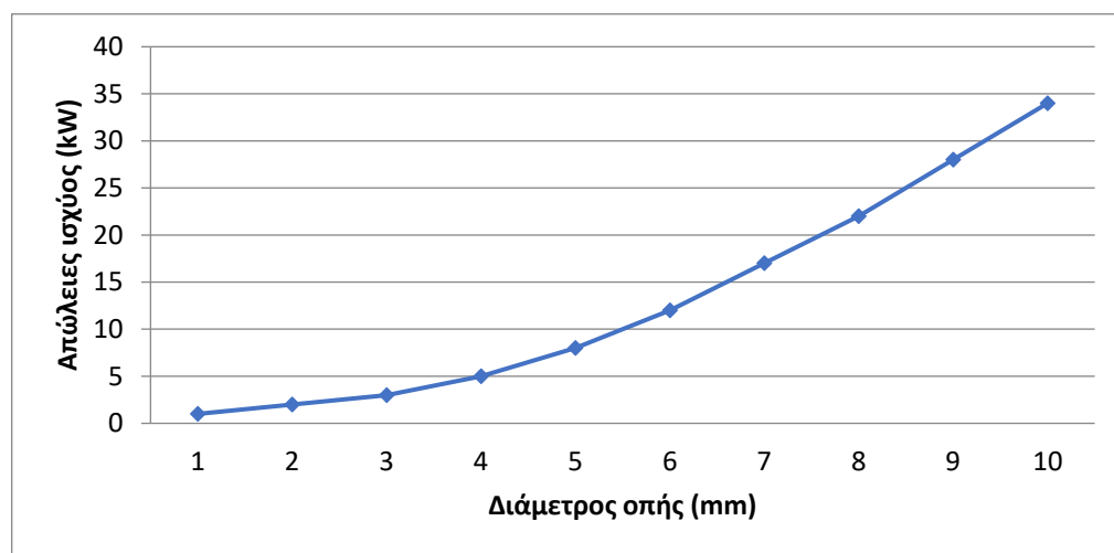
Σχήμα 1.10: Σχέση απωλειών ισχύος με διάμετρο οπής [23].
