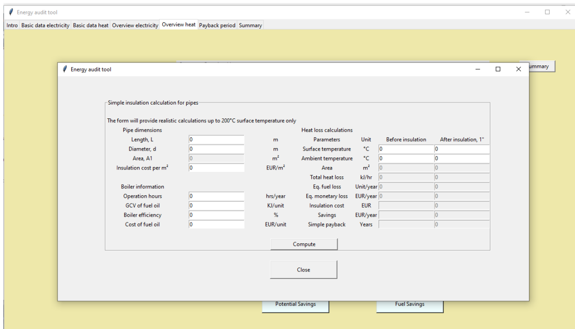
Σχήμα 2.23 : Καρτέλα υπολογισμού μόνωσης σωληνώσεων.
