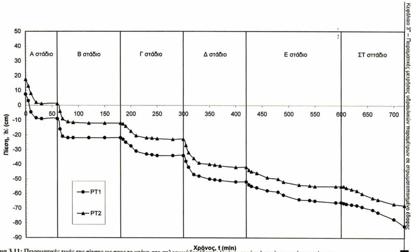
Σχήμα 3.11: Πειραματικές τιμές της πίεσης ως προς το χρόνο στο ηλιοαμμώδες έδαφος (επάνω στρώση) κατά την πρώτη στράγγιση
