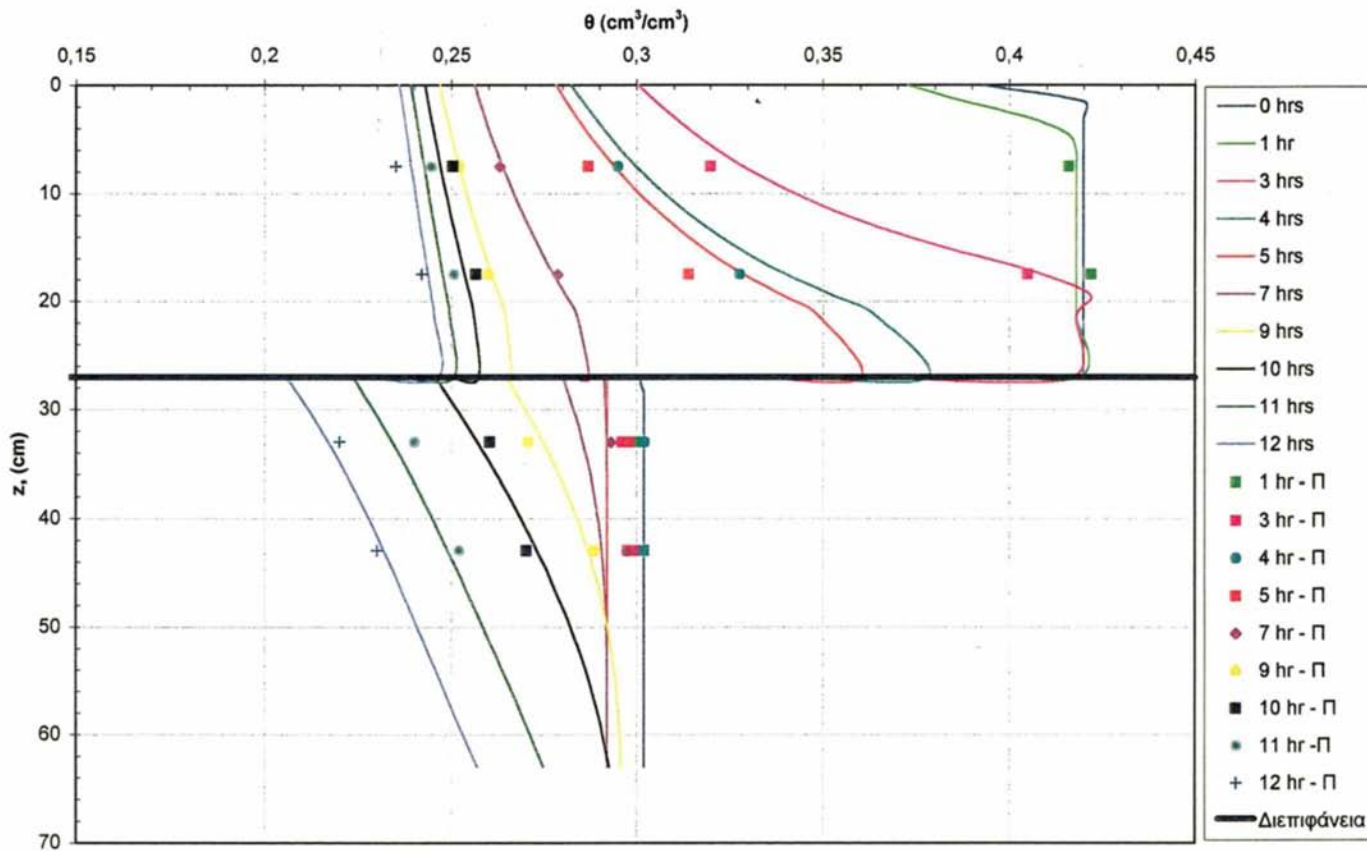
Σχήμα 6.11: Μέτωπα υγρασίας κατά την στράγγιση, με την συνεχή γραμμή η προσομοίωση, με τα σημεία οι πειραματικές τιμές όπως φαίνεται στο υπόμνημα, (μέθοδος Marquardt- σχέση Gardner).
