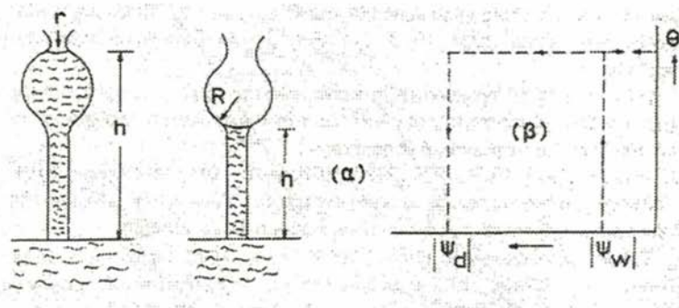
Σχήμα 1.7: Σχηματική παράσταση της θεωρίας του λαιμού φιάλης. (α) Υποθετική παράσταση πόρου γεμάτου και άδειου με νερό. (β) Βρόχος υστέρησης
