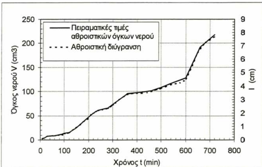
Σχήμα 6.6: Αθροιστική διύγρυνση
