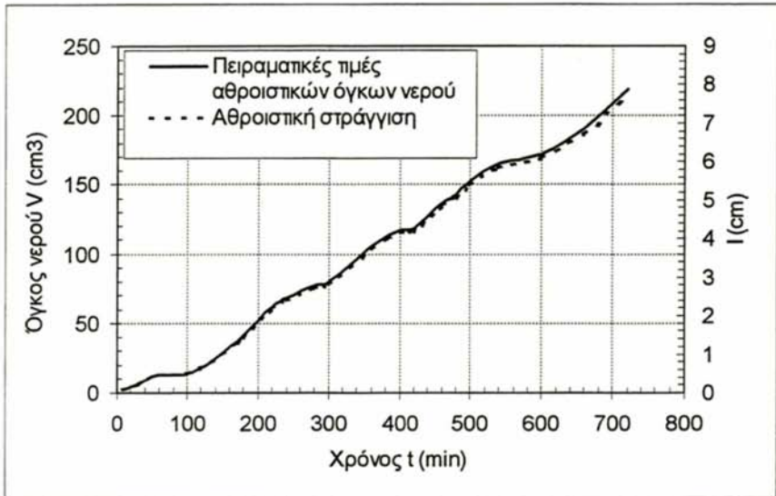
Σχήμα 6.5: Αθροιστική στράγγιση
