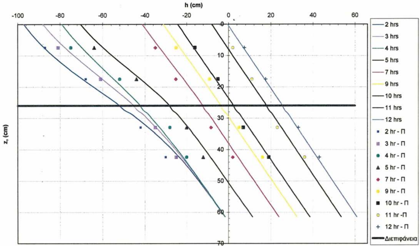
Σχήμα 6.10: Μέτωπα πίεσης κατά την δώγρανση, με την συνεχή γραμμή η προσομοίωση, με τα σημεία οι πειραματικές τιμές όπως φαίνεται στο υπόμνημα, (μέθοδος συζυγών- σχέση Gardner).
