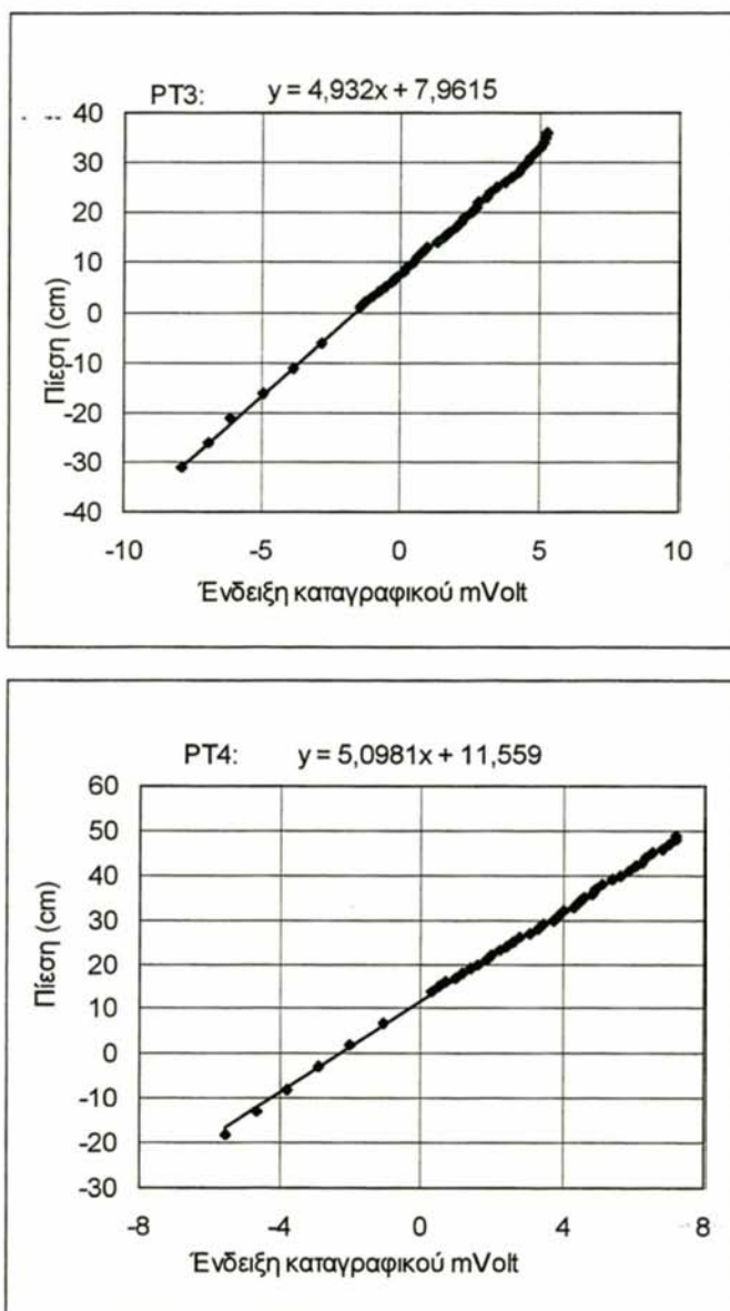
Σχήμα 3.2β: Καμπύλες βαθμονόμησης των μετατροπέων πίεσης
