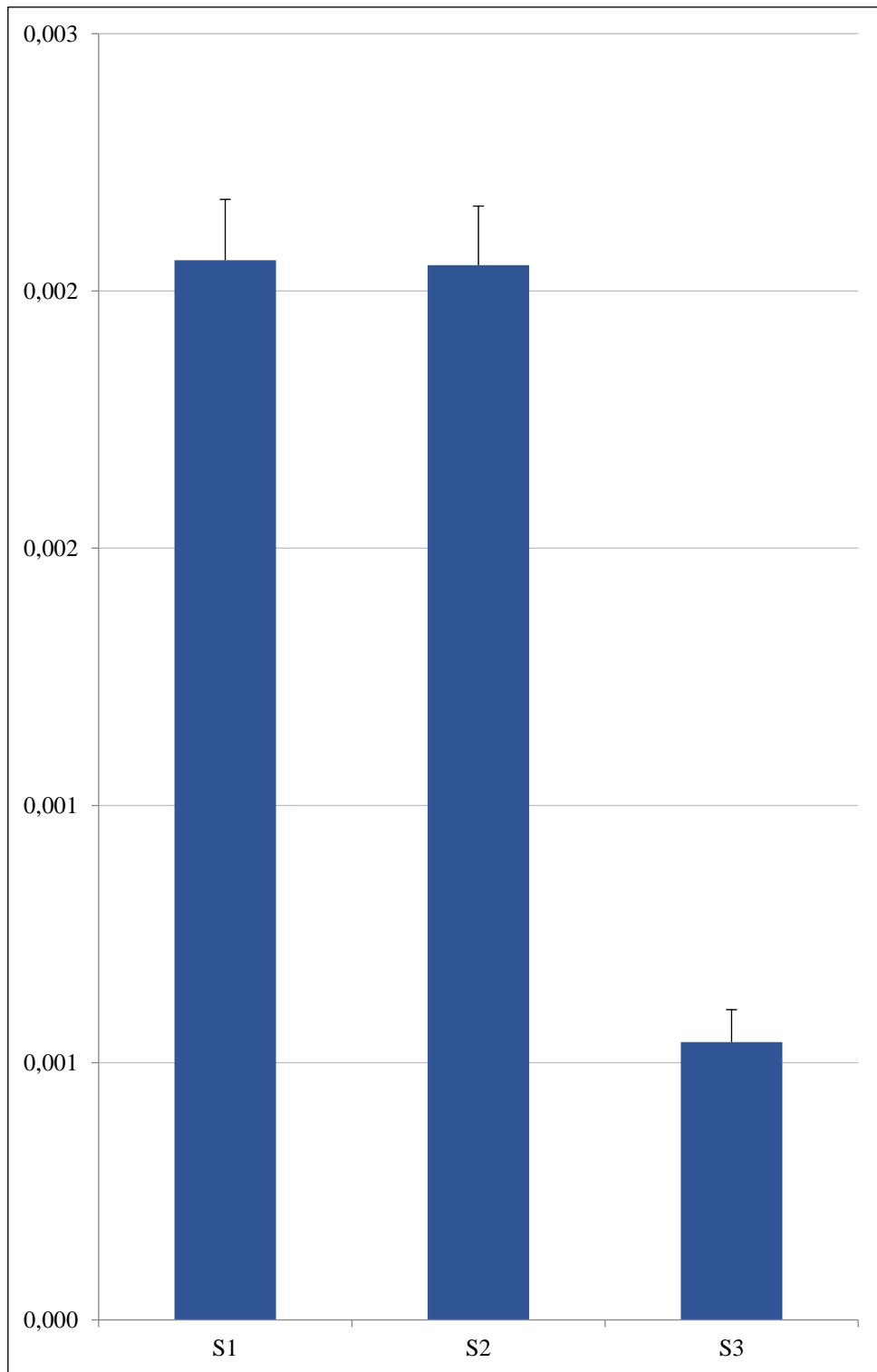
Σχήμα 3.17: Διάγραμμα με τη μέση τιμή και την τυπική απόκλιση των νιτρικών (µM) στους 3 σταθμούς δειγματοληψίας.
