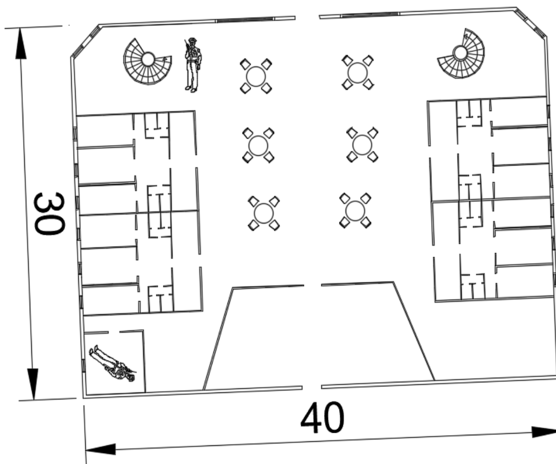
Εικόνα 6: Κάτοψη Ισογείου
