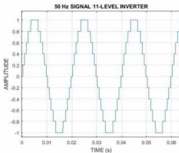
Εικόνα 3.36 Η κυματομορφή συχνότητας 50 Hz φασικής τάσης εξόδου πολυβάθμιου αντιστροφέα έντεκα επιπέδων με τη μέθοδο HH.
