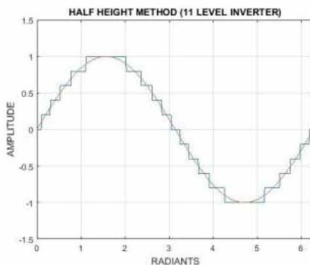
Εικόνα 3.35 Η προκύπτουσα κυματομορφή με εφαρμογή της μεθόδου HH για πολυβάθμιο αντιστροφέα έντεκα επιπέδων.
