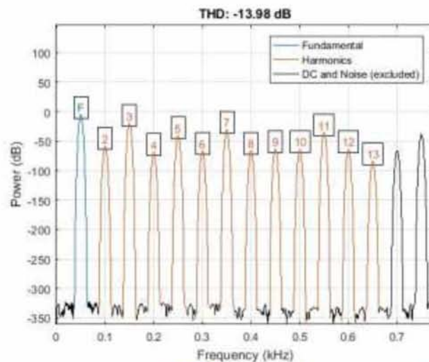
Εικόνα 3.19 Φάσμα της κυματομορφής 50HZ που προκύπτει με τη μέθοδο EP για πολυβάθμιο αντιστροφέα έντεκα επιπέδων.
