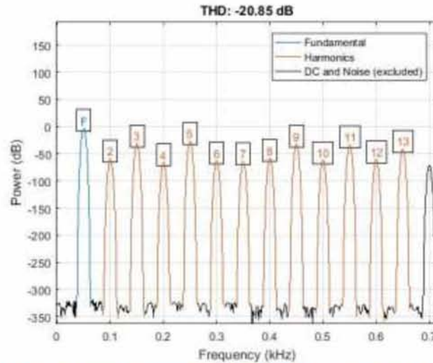
Εικόνα 3.4 Φασματικό περιεχόμενο της κυματομορφής εξόδου του πολυβάθμιου αντιστροφέα επτά επιπέδων.
