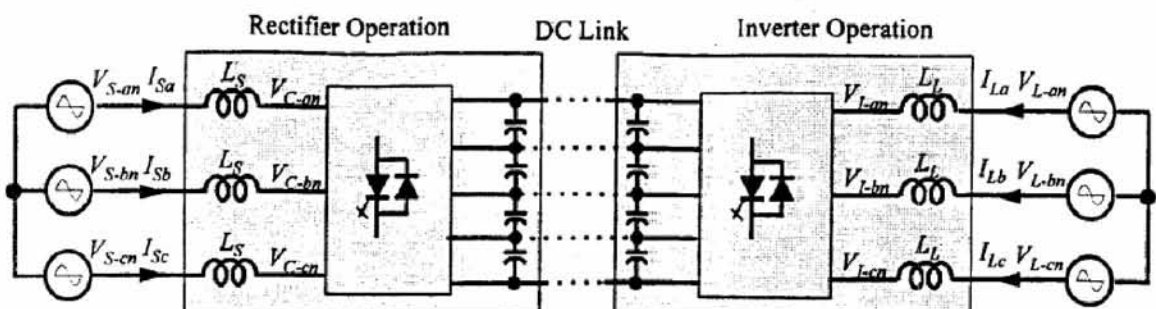
Εικόνα 1.12 Πολυβάθμιοι μετατροπείς συνδεδεμένοι σε διάταξη Back to Back Intertie.
