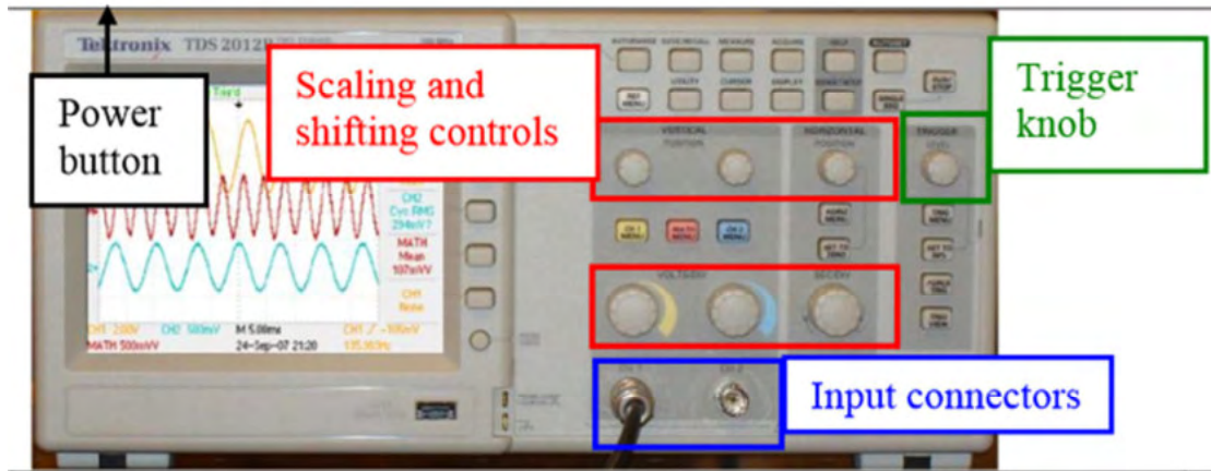
Εικόνα 3: Πρόσοψη παλμογράφου Tektronix TDS 2012B
