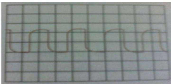
Εικόνα 22: φαινόμενο υποαντιστάθμισης
