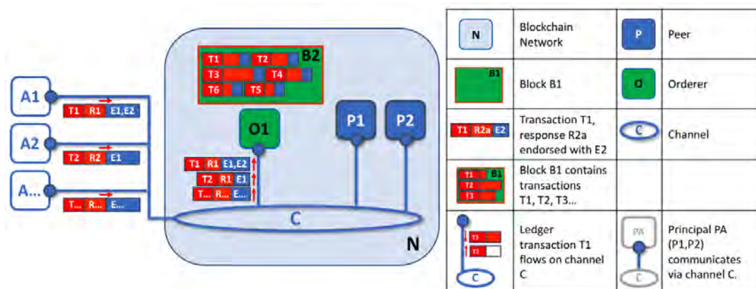
Σχήμα 3.12: Το δεύτερο στάδιο της συναλλαγής στο Hyperledger Fabric (2017)
