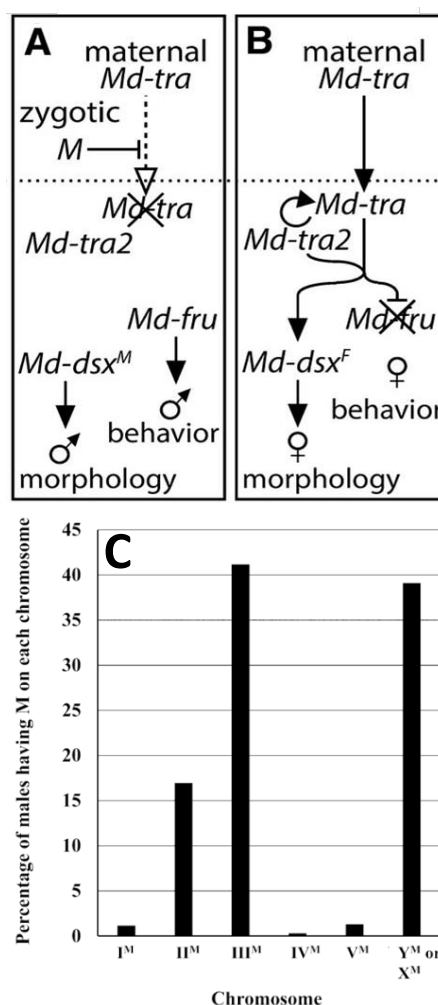
Εικόνα 8. Το Μονοπάτι φυλοκαθορισμού και ο παράγοντας M στην οικιακή μύγα Musca domestica . A: μονοπάτι προς ανάπτυξη αρσενικού. B: μονοπάτι προς ανάπτυξη θηλυκού. C: Ποσοστά αρσενικών που φέρουν τον παράγοντα M σε κάθε ένα από τα χρωμοσώματα.
