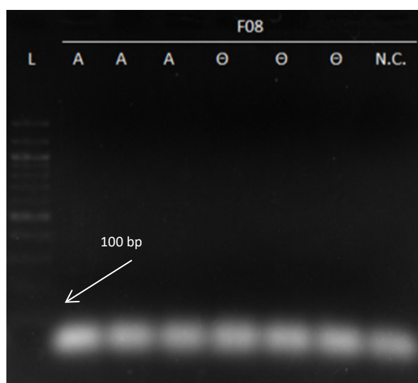
Εικόνα 25. Ηλεκτροφόρηση σε πήκτωμα αγαρόζης 1,5% των προϊόντων της PCR με το ζεύγος εκκινητών F08. Μέγεθος προϊόντος 120bp. Παρατηρούμε την απουσία αυτού του προϊόντος. A: Αρσενικό, Θ: θηλυκό, N.C.: Αρνητικός μάρτυρας, L: μάρτυρας μεγεθών.
