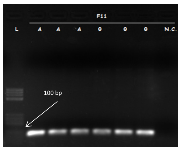
Εικόνα 25. Ηλεκτροφόρηση σε πήκτωμα αγαρόζης 1,5% των προϊόντων της PCR με το ζεύγος εκκινητών F11. Μέγεθος προϊόντος 104bp. Παρατηρούμε την ενίσχυση του ίδιου προϊόντος σε αρσενικά και θηλυκά. A: Αρσενικό, Θ: θηλυκό, N.C.: Αρνητικός μάρτυρας, L: μάρτυρας μεγεθών.
