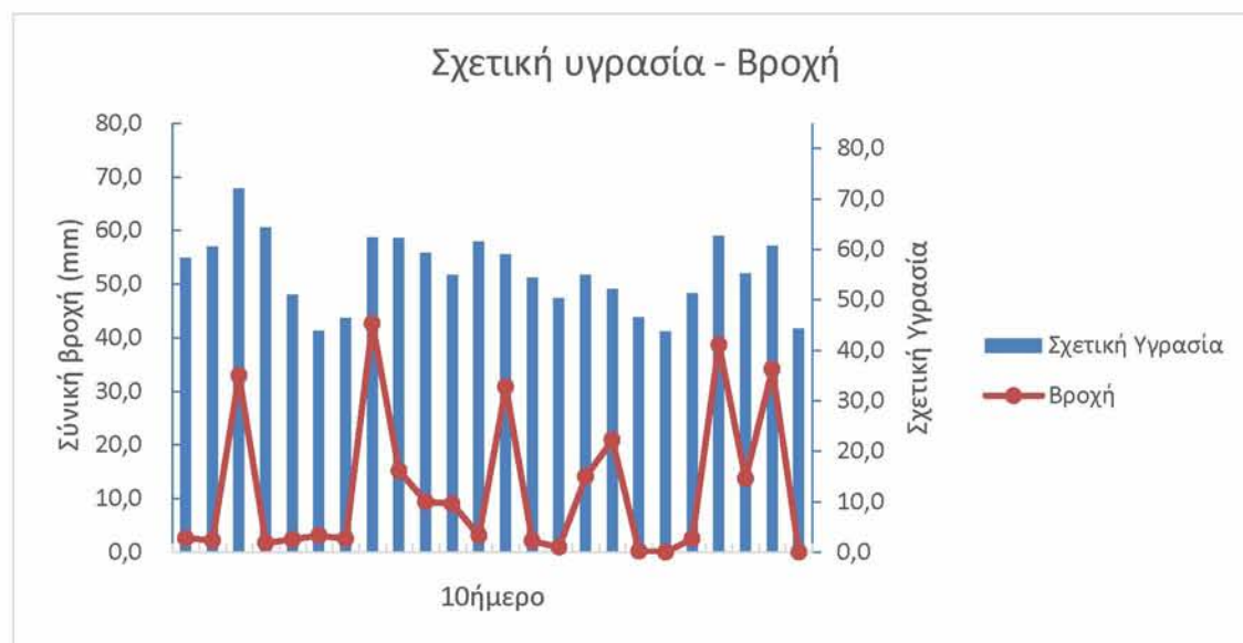
Γράφημα 2. Μέσες τιμές σχετικής υγρασίας(%) και άθροισμα βροχοπτώσεων(mm) ανά δεκάημερο από τους μήνες Νοέμβριος 2016 έως Ιούνιος 2017.
