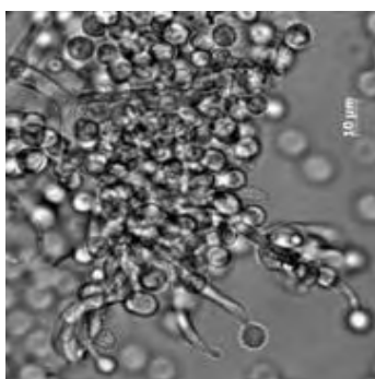
Εικόνα 17. F. Langsethiae
