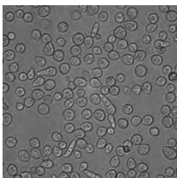
Εικόνα 16. F. Sporotrichioides
