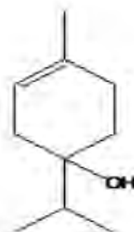
Τερπινεν-4-όλη
